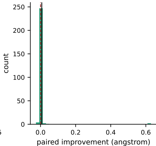
RMSD
