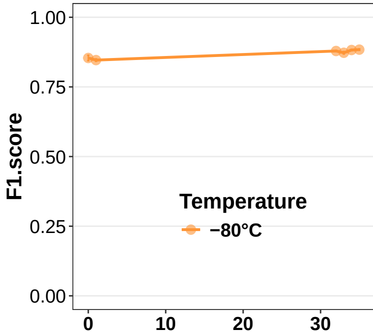
InDels
