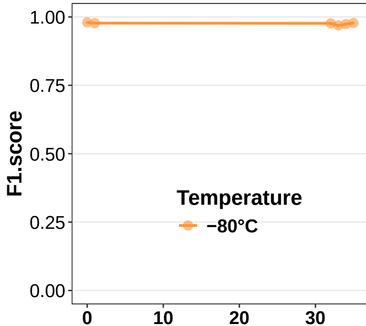
SNVs
