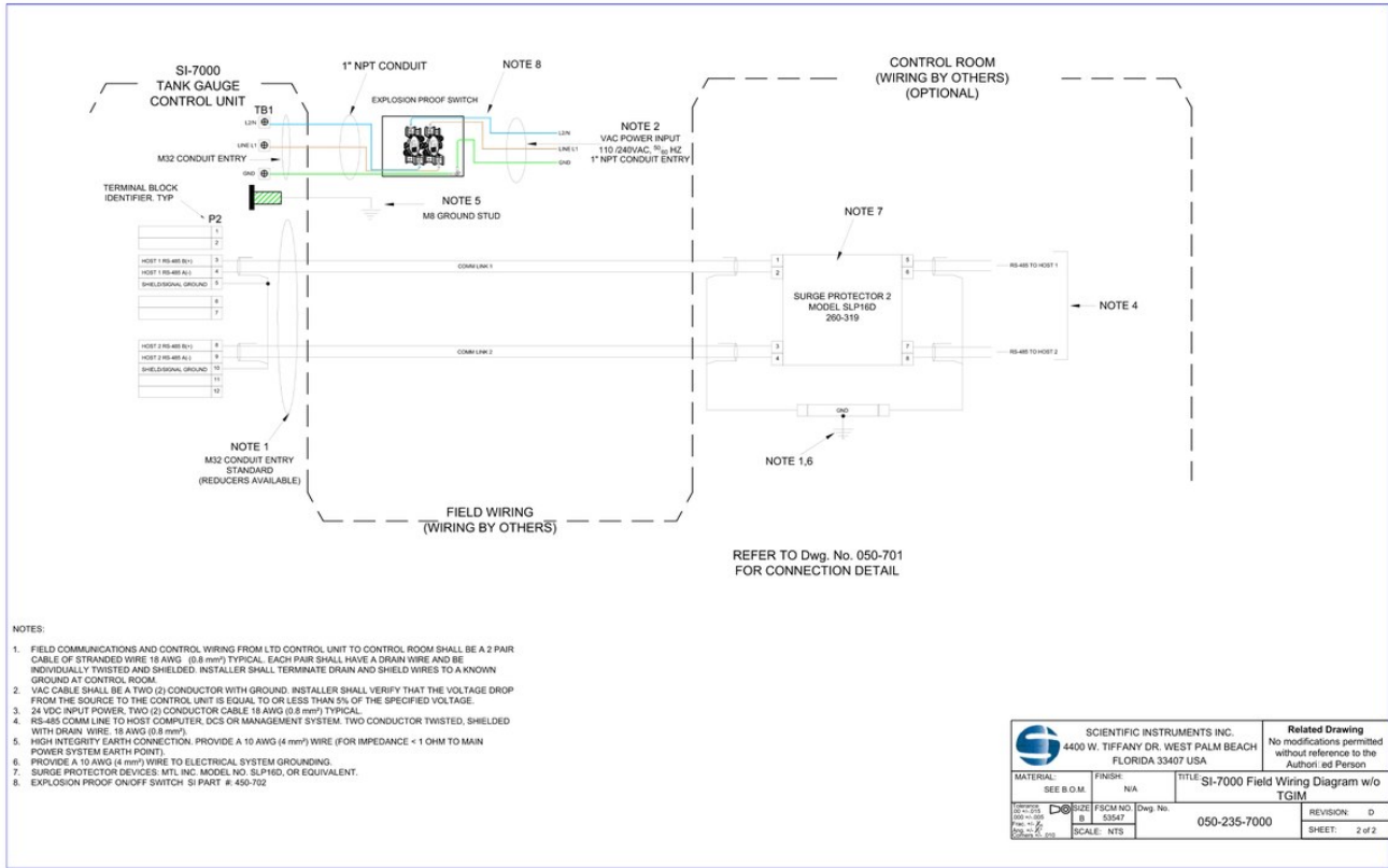
SI-7000 不带 TGIM 的现场接线图
