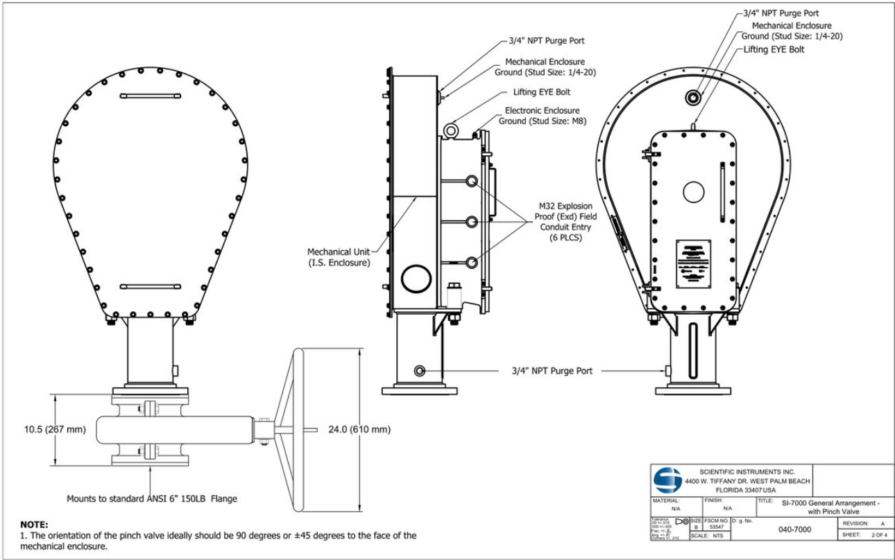
SI-7000 带 Pinch Valve 布置图 Sheet 2
