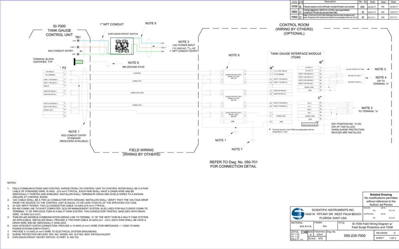
SI-7000 带现场浪涌保护和 TGIM 的现场接线图
