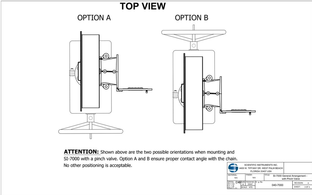
SI-7000 带 Pinch Valve 顶视方向图 Sheet 3
