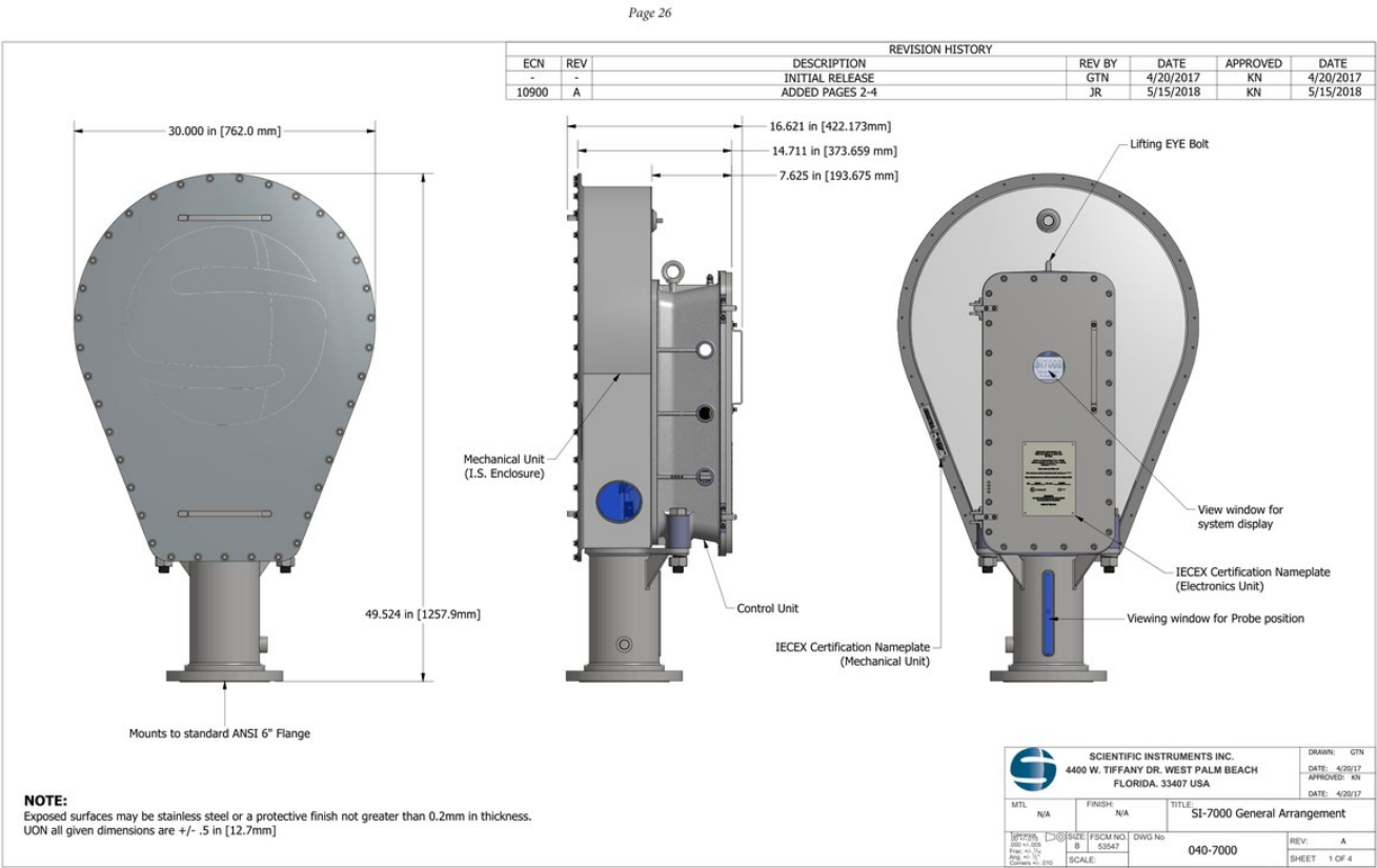
SI-7000 总体布置图 Sheet 1
