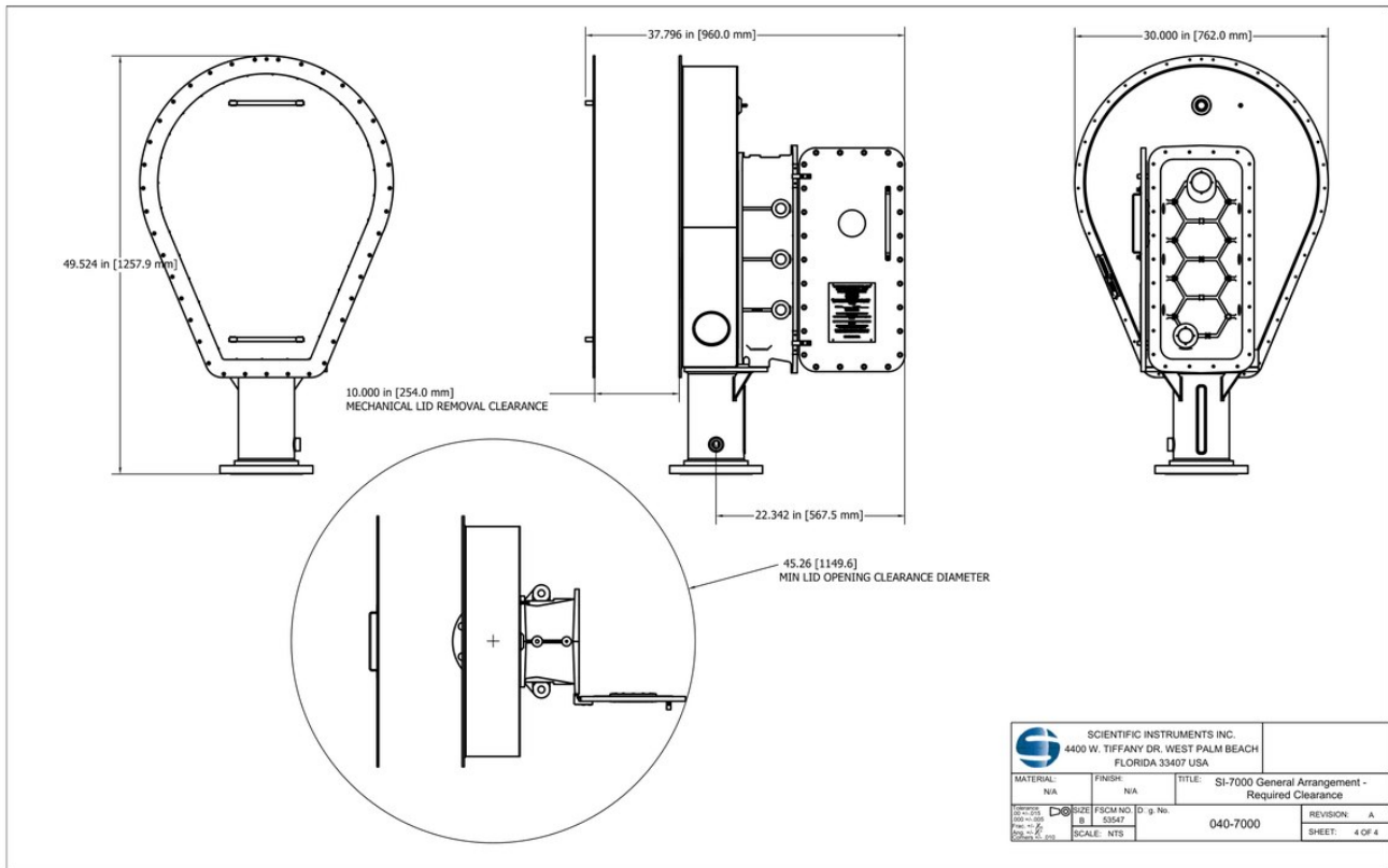
SI-7000 所需间隙图 Sheet 4
