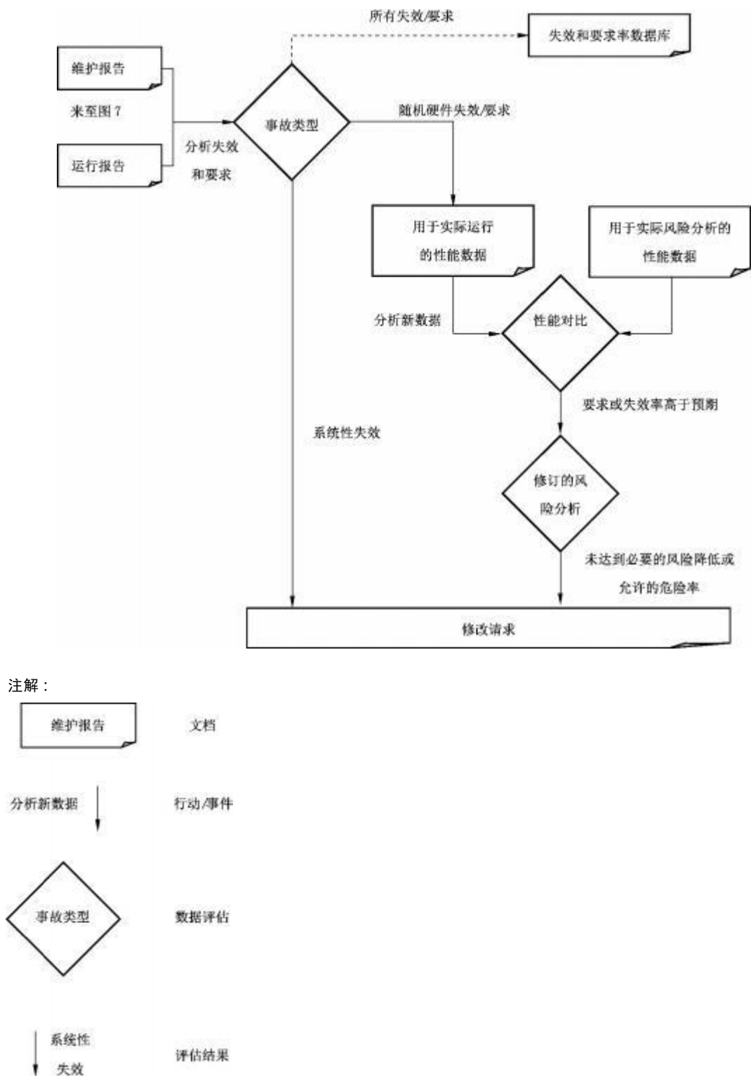
图 8 运行和维修管理模型示例
