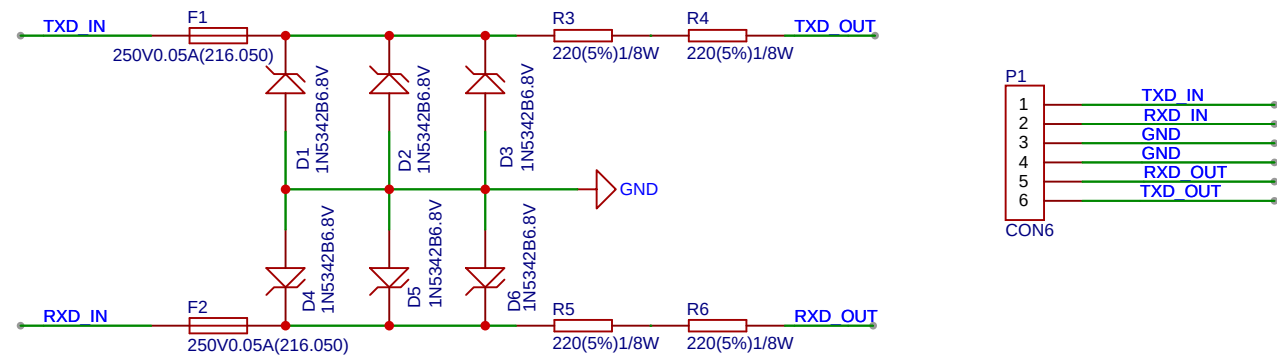
信号安全栅原理图
