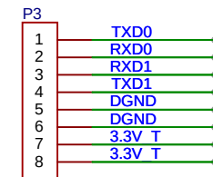
RTD板间接口
