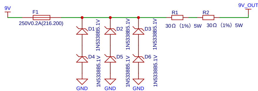
电源安全栅原理图
