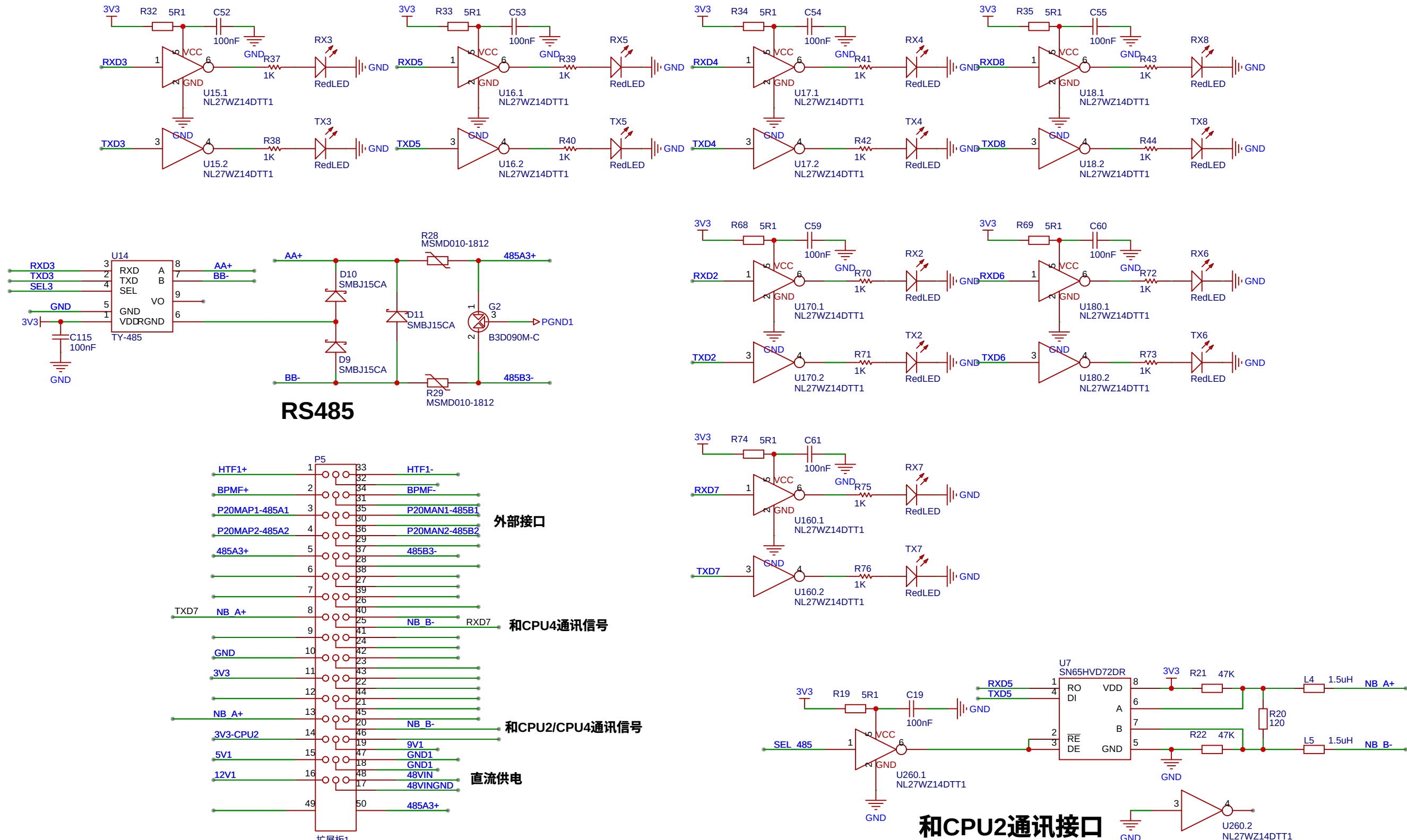
SIL-MAIN主板原理图
