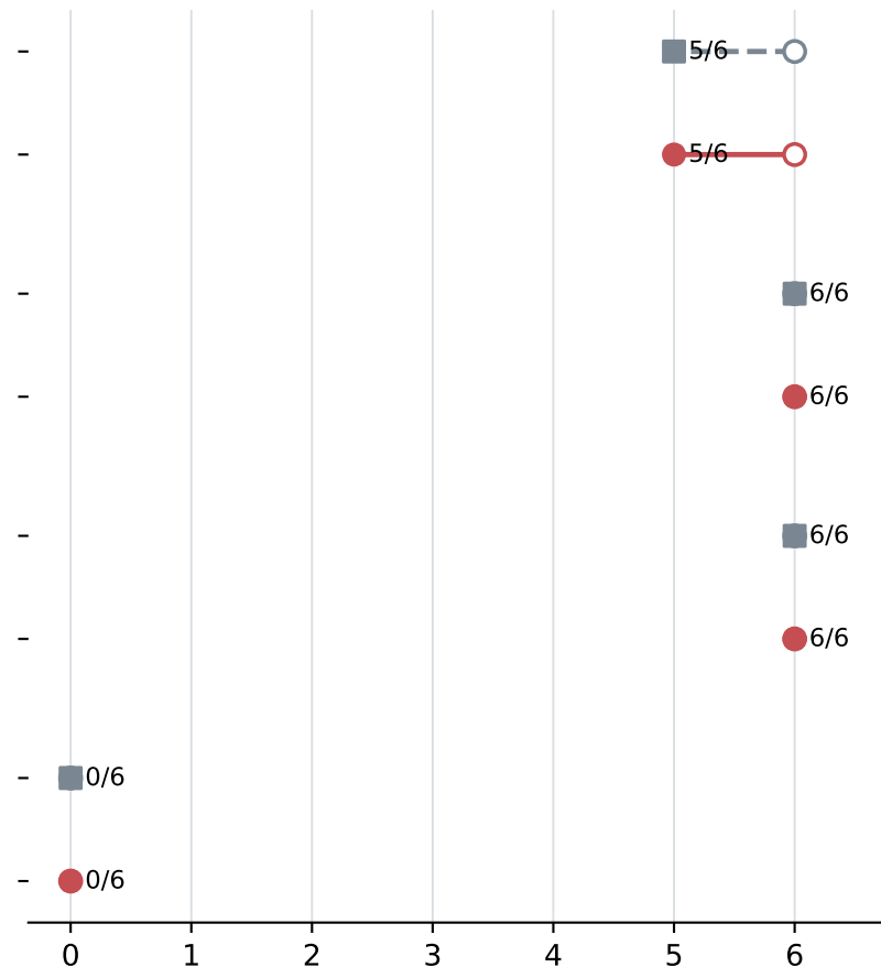
Layer 24
