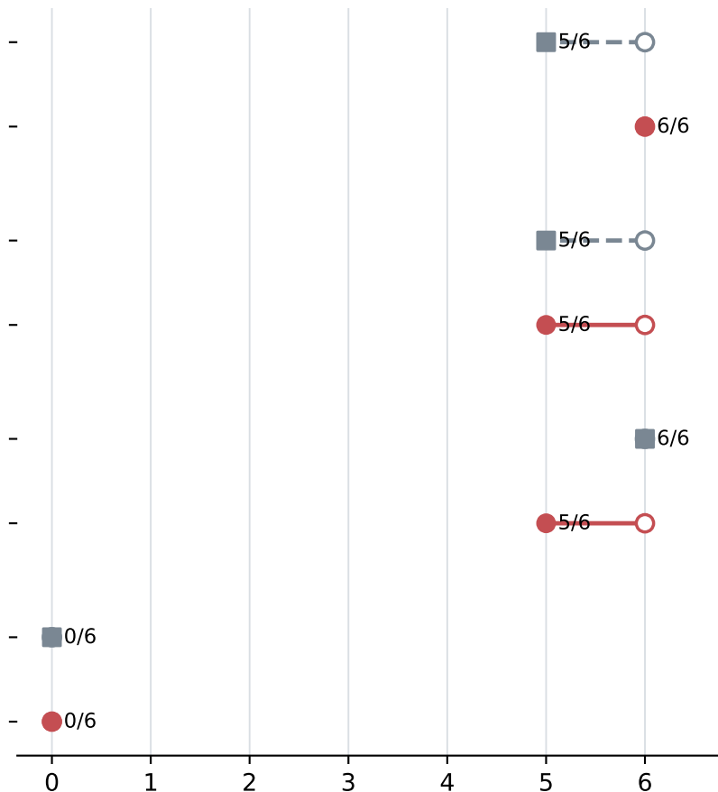
Layer 8
