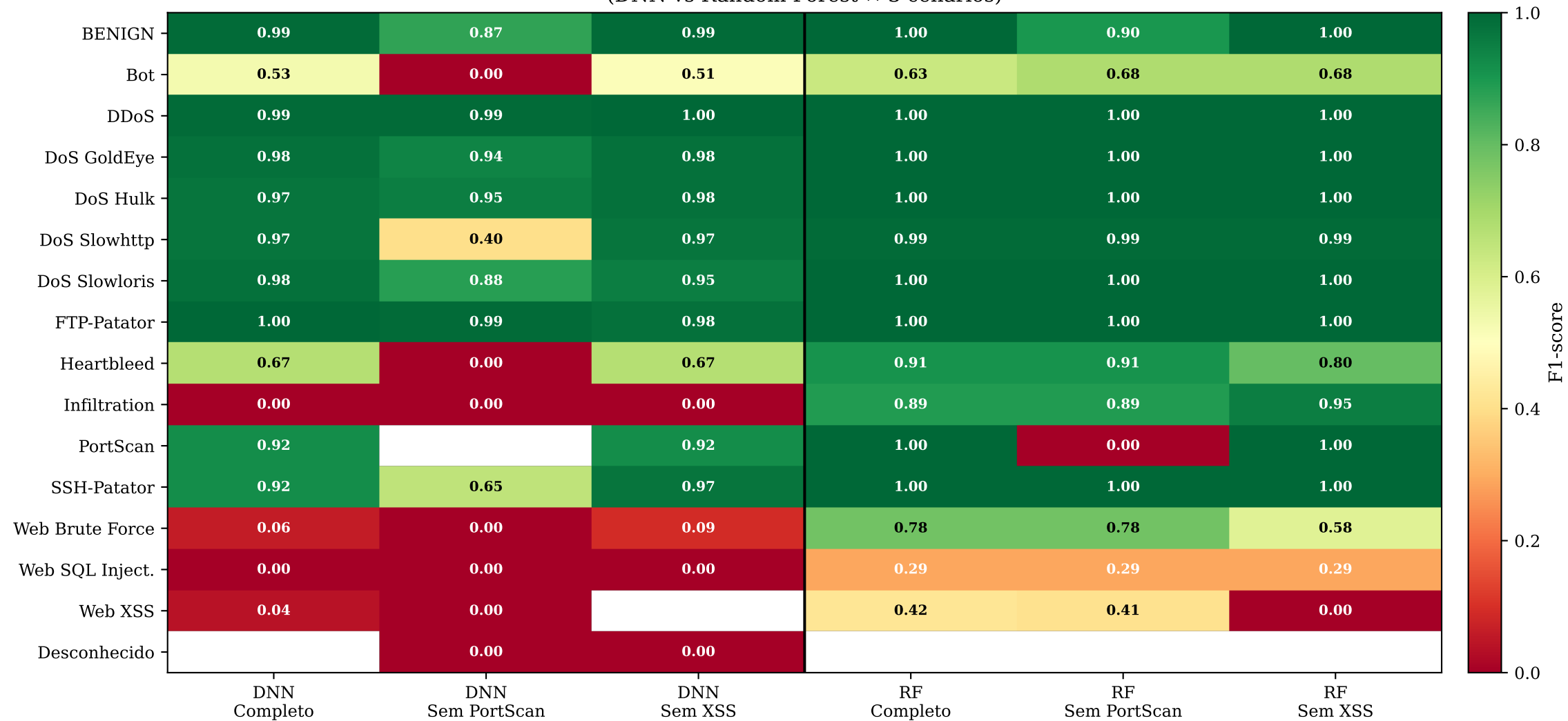
Heatmap de F1-score por Classe — Baseline CICIDS2017 (DNN vs Random Forest × 3 cenários)
