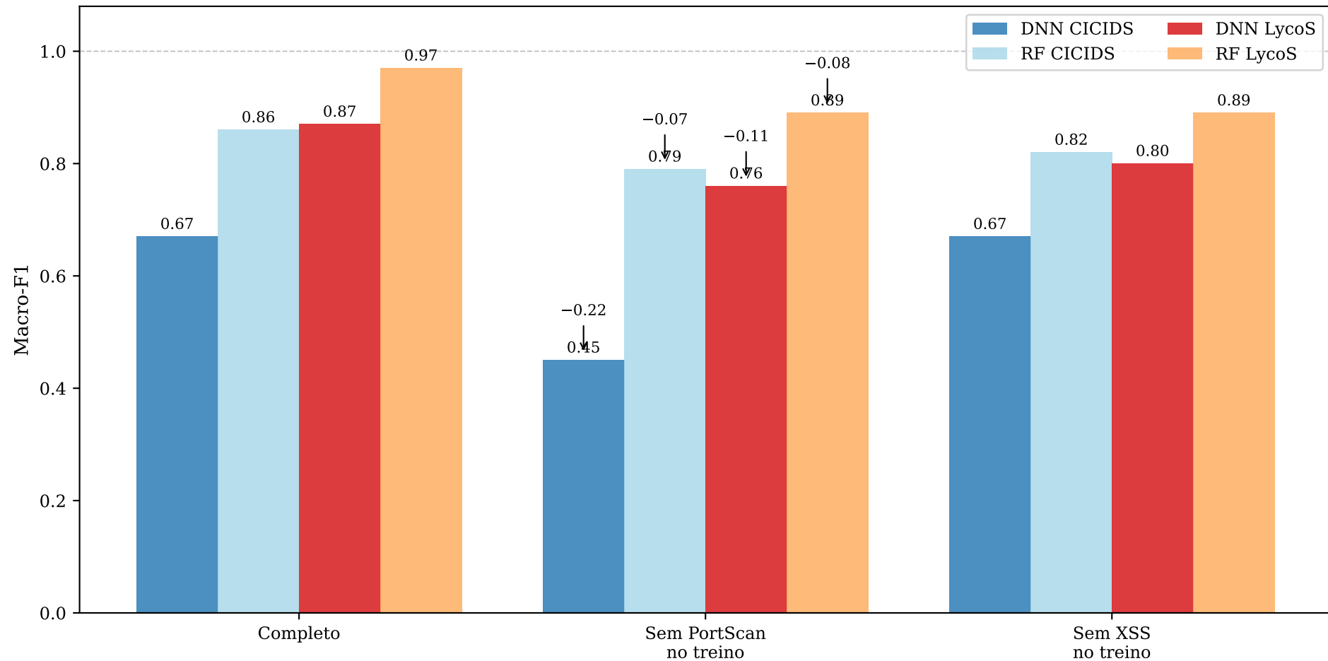
Degradação de Macro-F1 por Cenário (Open-Set Generalization) CICIDS2017 e LycoS-IDS2017
