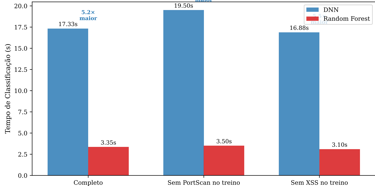
Tempo de Inferência — DNN vs Random Forest (CICIDS2017, conjunto de teste)
