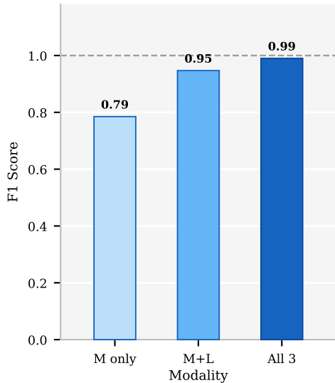
RQ1: Detection F1
