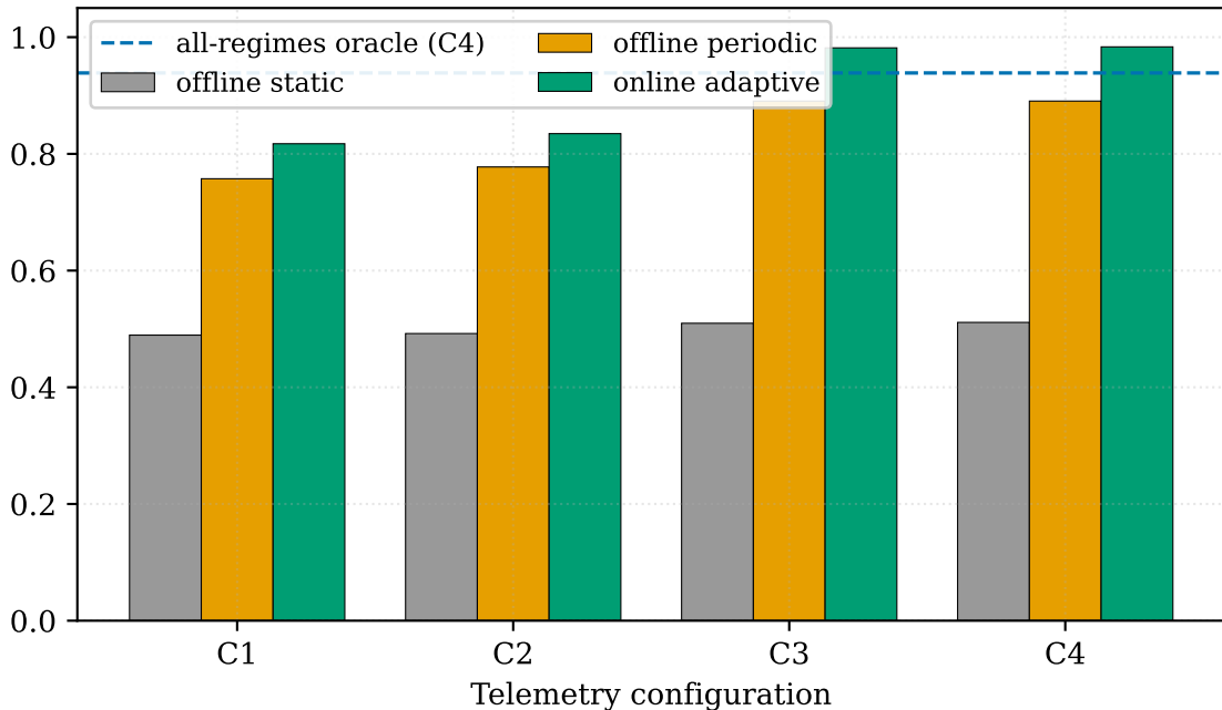
F1 on drifted future stream
