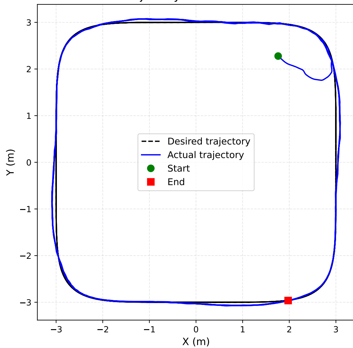
2D Trajectory: Desired vs Actual
