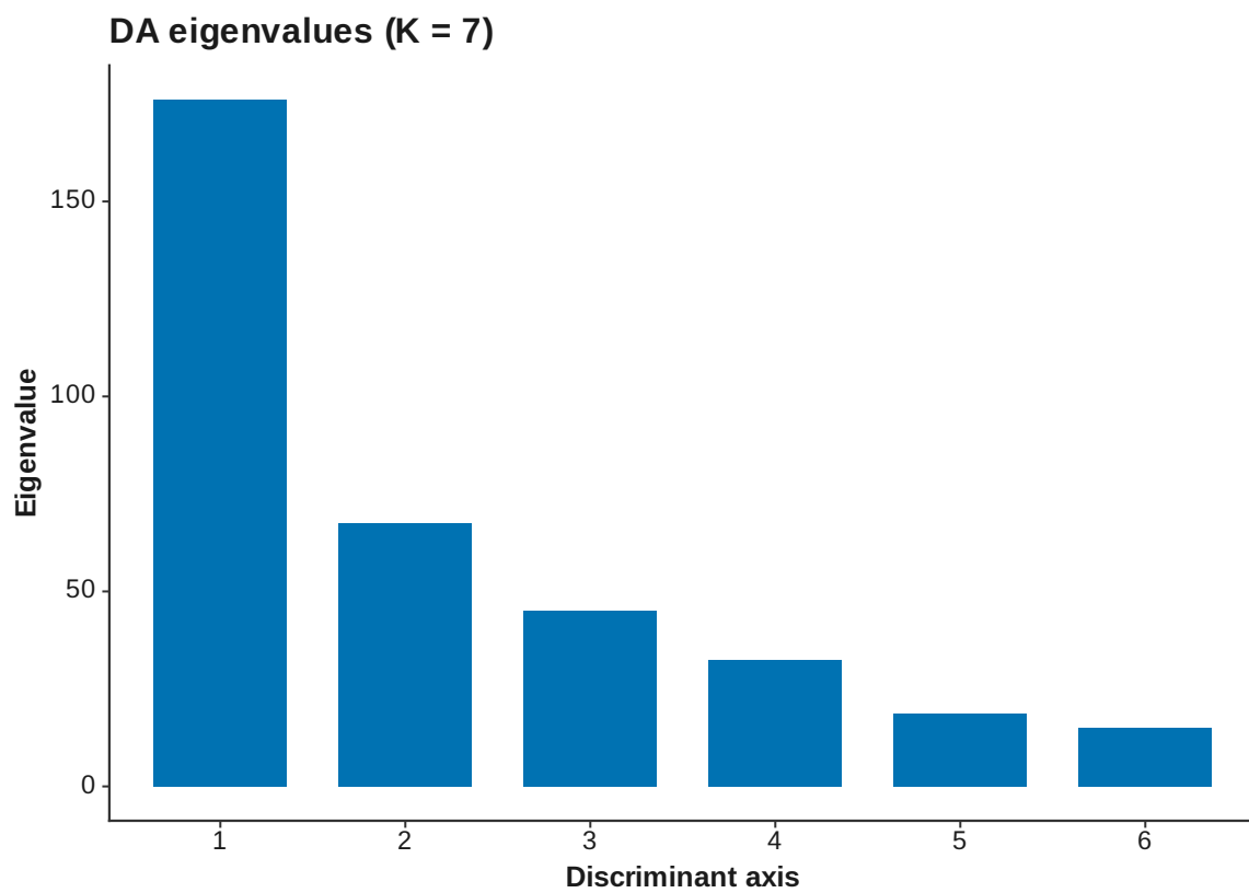
Figure 38: DAPC eigenvalues K 7
