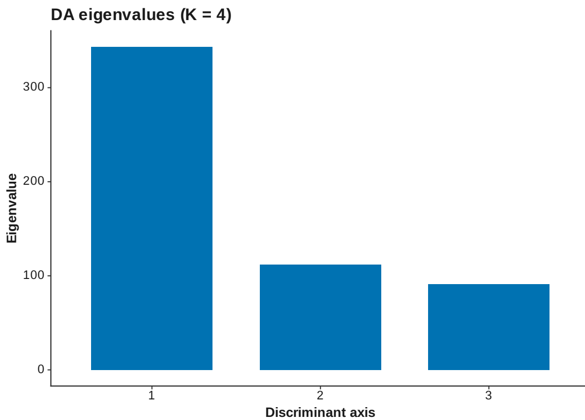
Figure 35: DAPC eigenvalues K 4
