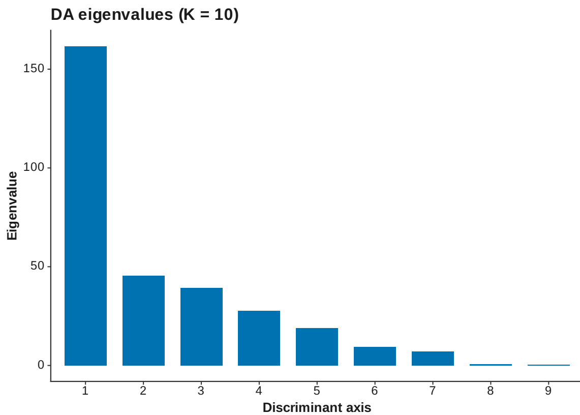
Figure 41: DAPC eigenvalues K 10
