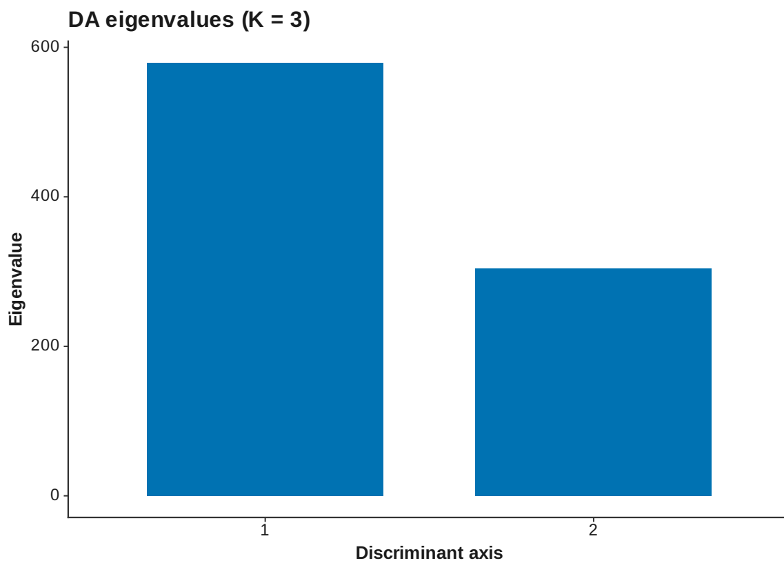
Figure 34: DAPC eigenvalues K 3
