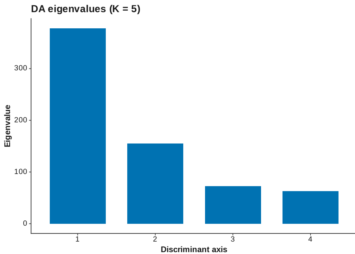
Figure 36: DAPC eigenvalues K 5
