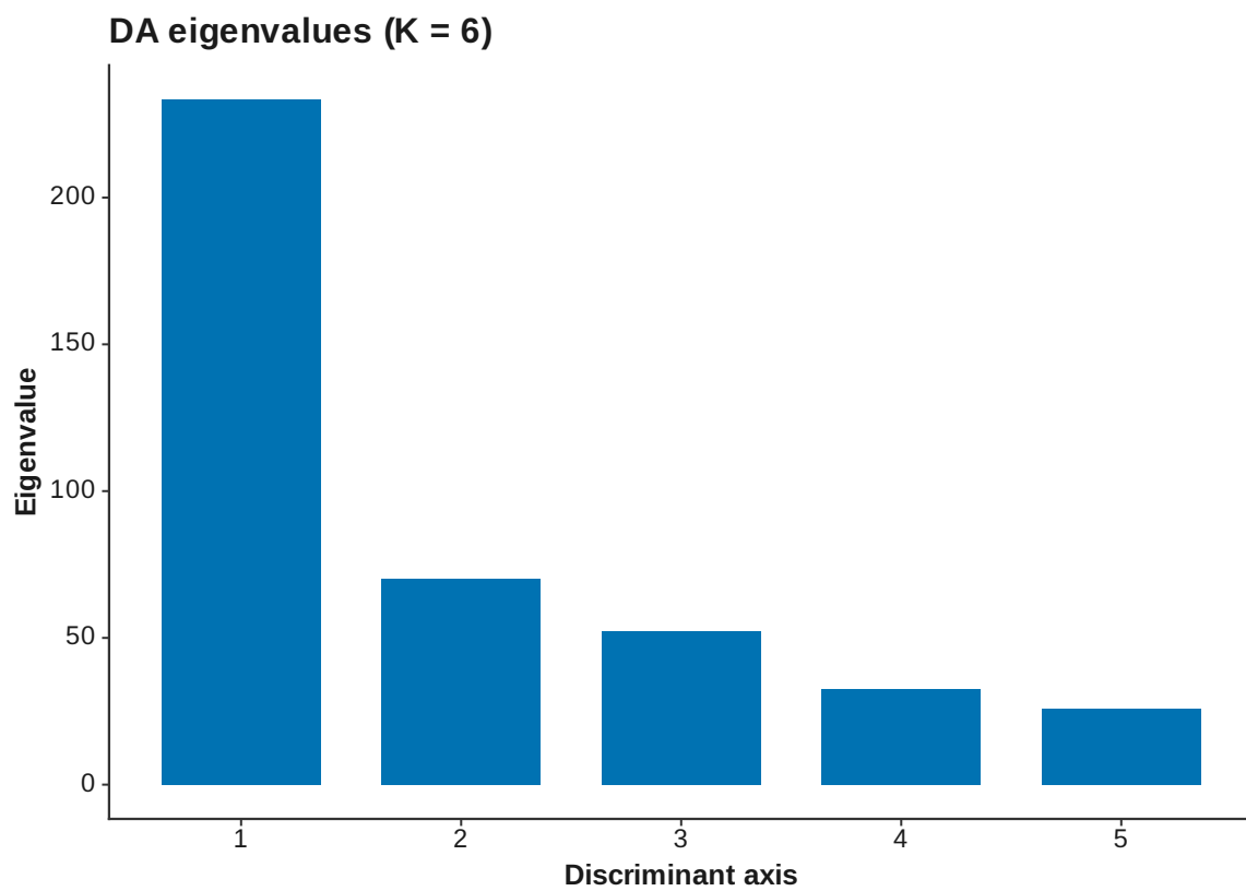
Figure 37: DAPC eigenvalues K 6
