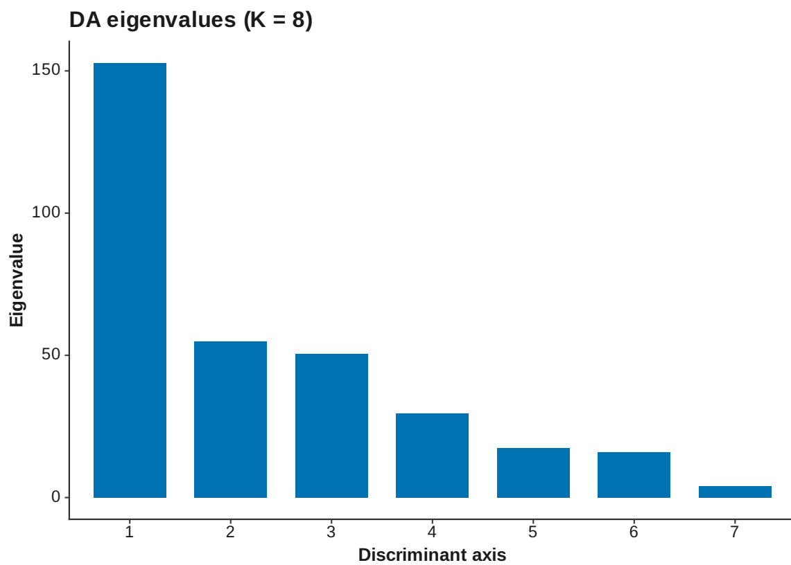
Figure 39: DAPC eigenvalues K 8
