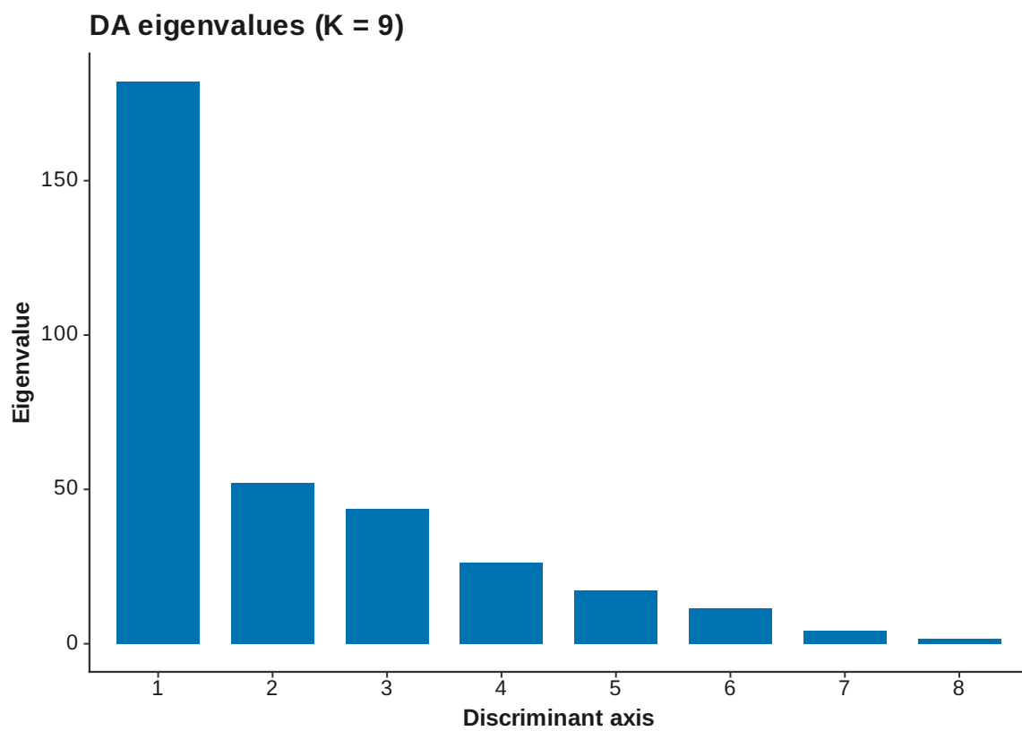
Figure 40: DAPC eigenvalues K 9
