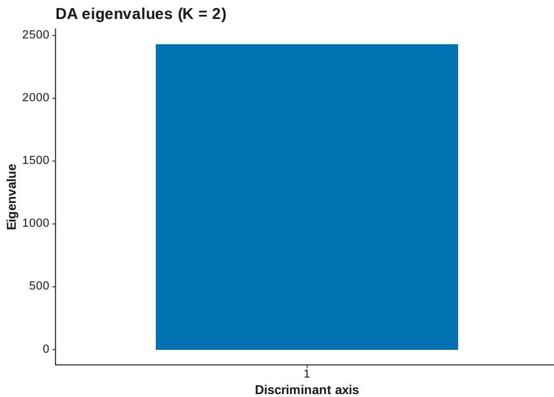
Figure 33: DAPC eigenvalues K 2
