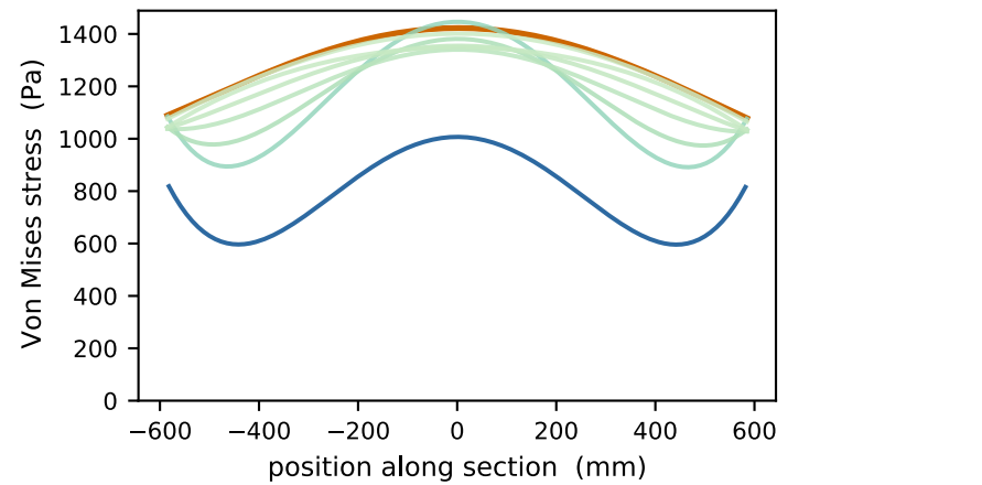
Motif 2 — section stress ( y=0 plane)
