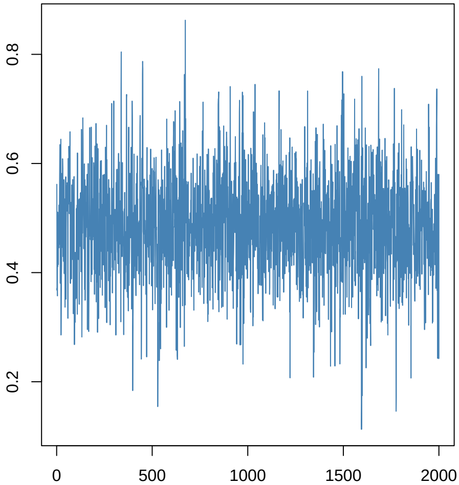
logTotLen_raw~logTotGenes_raw
