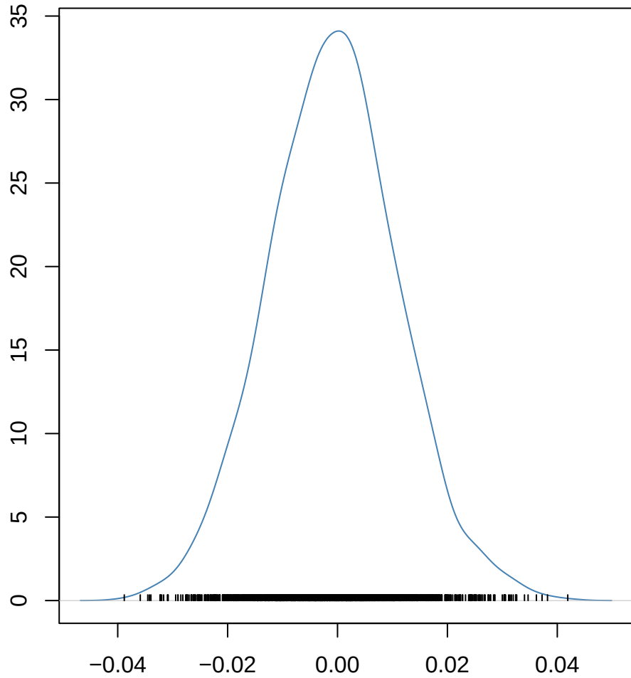
logTotGenes_raw~masdif
