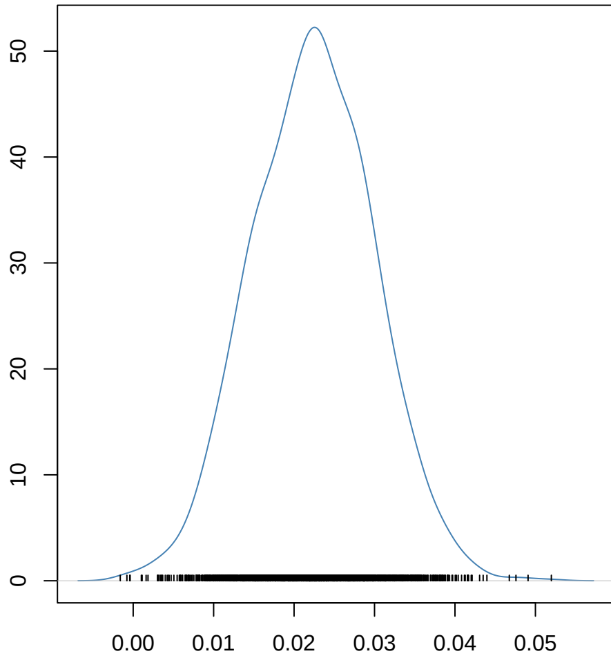
logTotLen_raw~masdif
