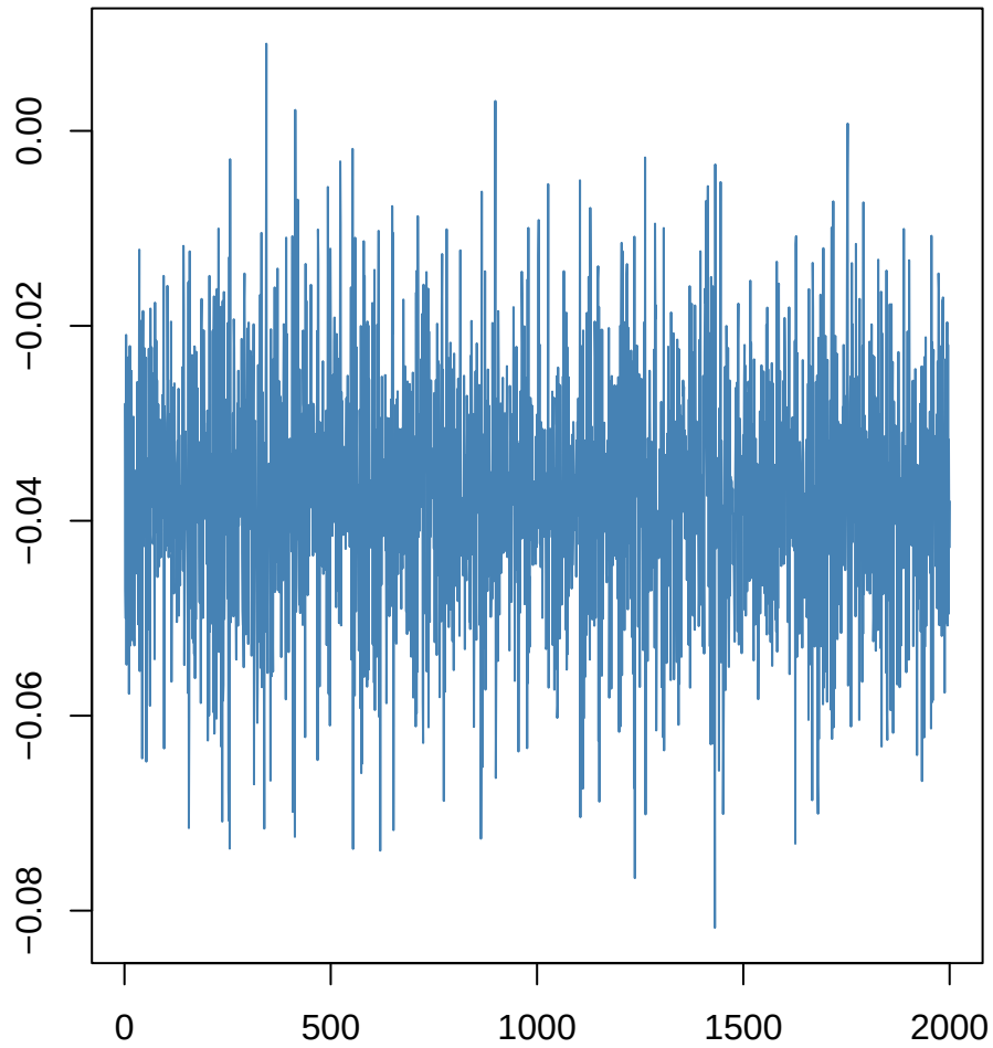
propAccelDn~masdif
