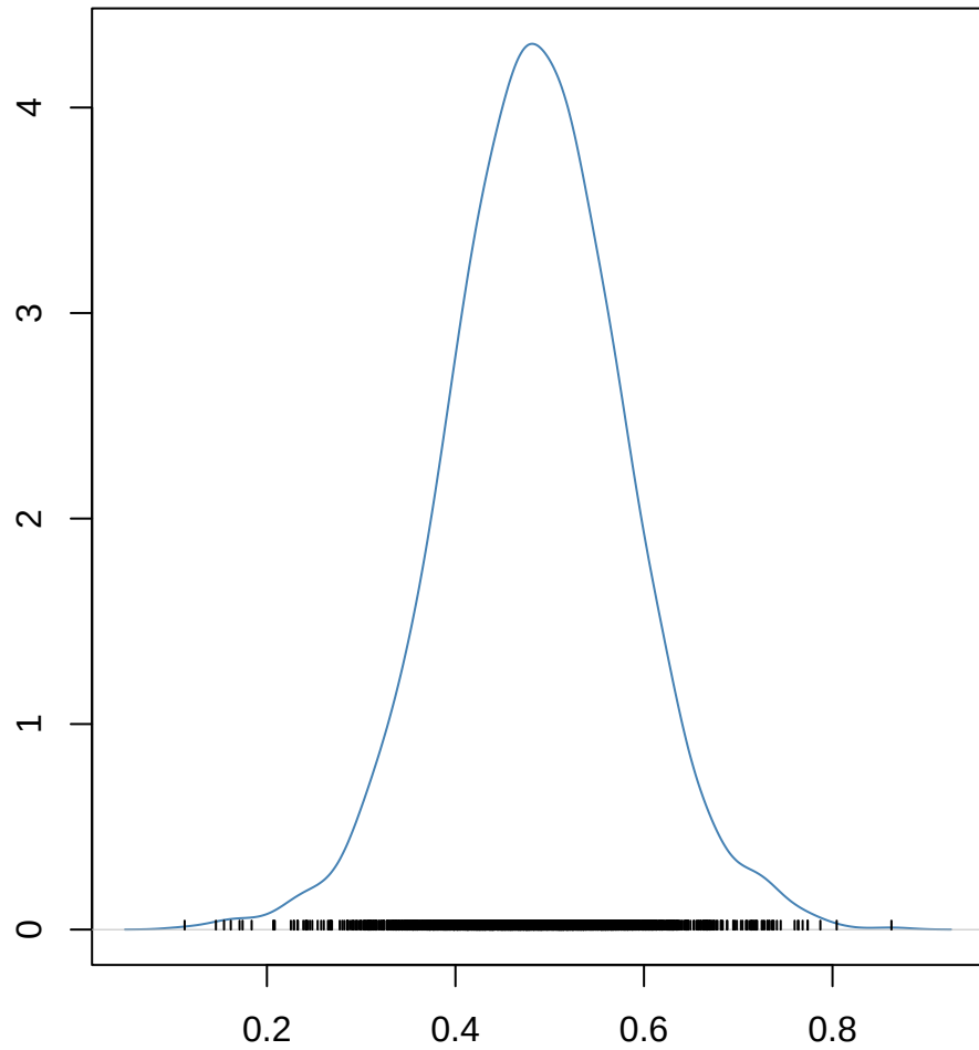
logTotLen_raw~logTotGenes_raw
