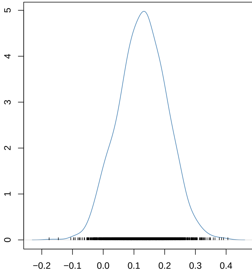
logTotLen_raw~propAccelDn
