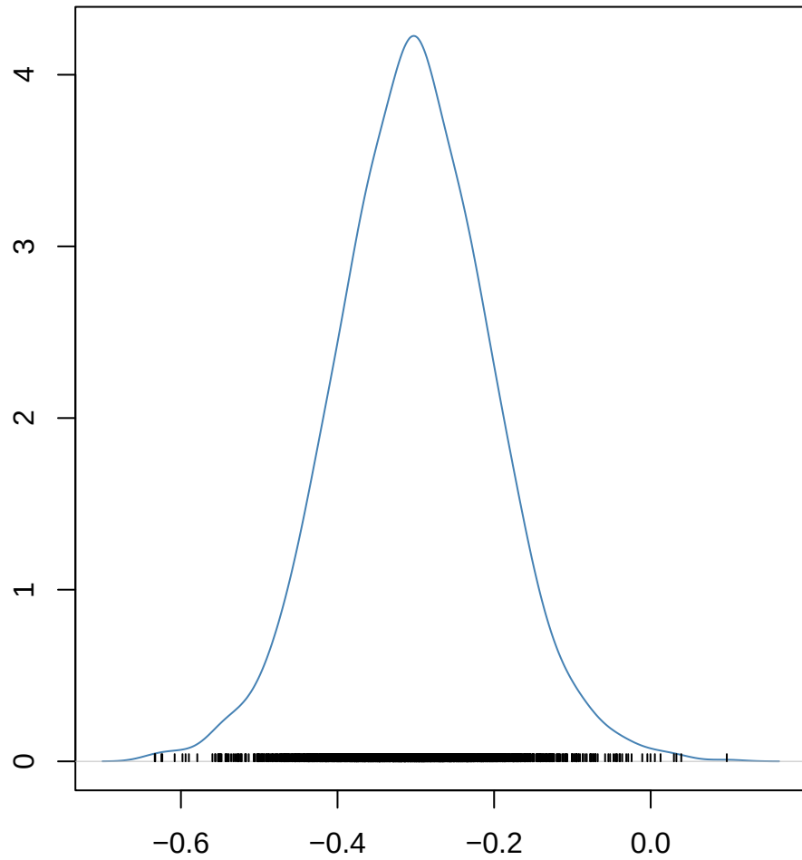
logTotLen_raw~logBUSCO
