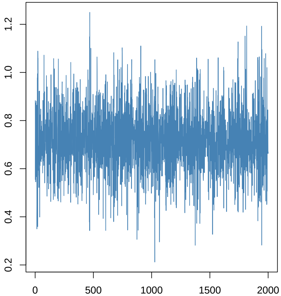
logTotGenes_raw~logBUSCO
