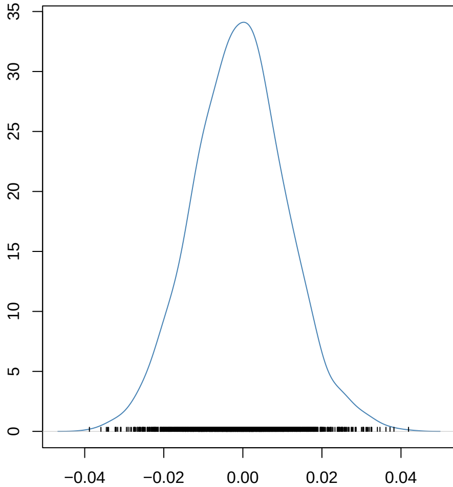
logTotGenes_raw~masdif
