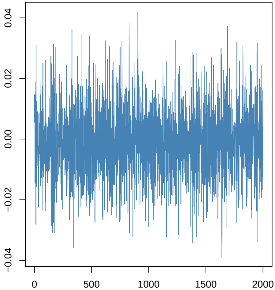
logTotGenes_raw~masdif
