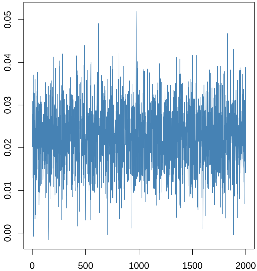
logTotLen_raw~masdif
