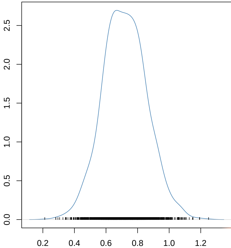
logTotGenes_raw~logBUSCO
