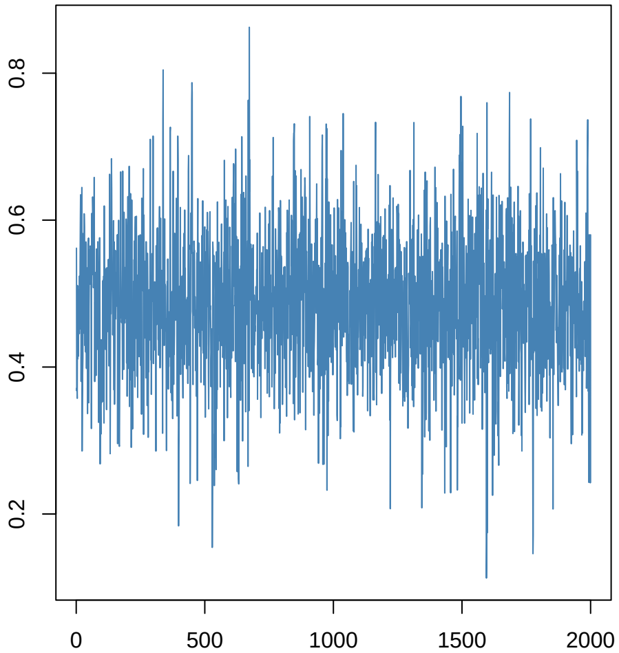
logTotLen_raw~logTotGenes_raw
