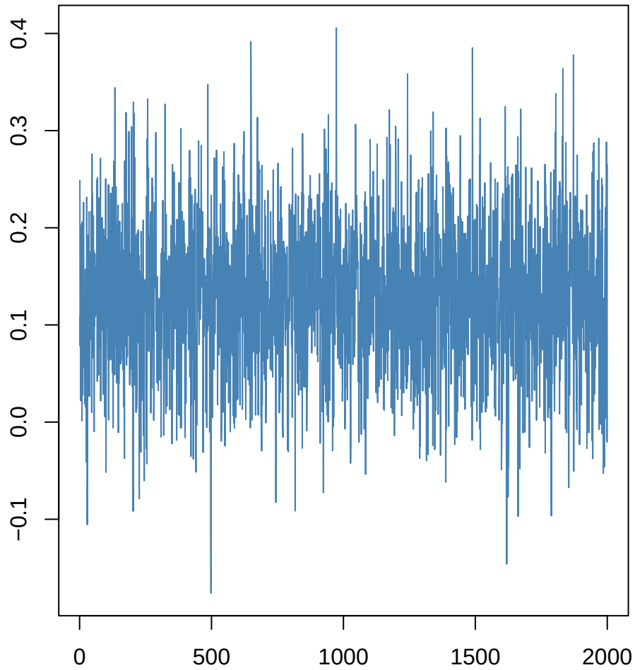
logTotLen_raw~propAccelDn
