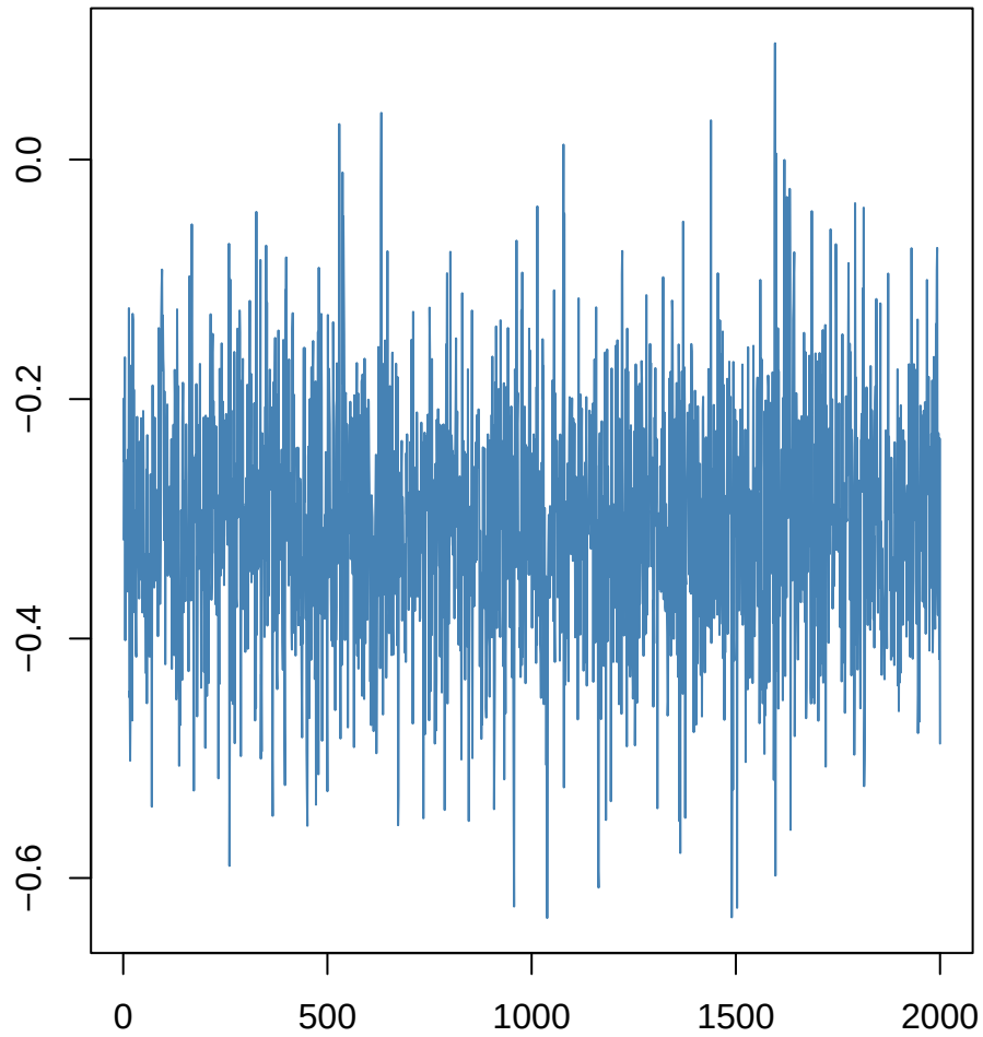
logTotLen_raw~logBUSCO
