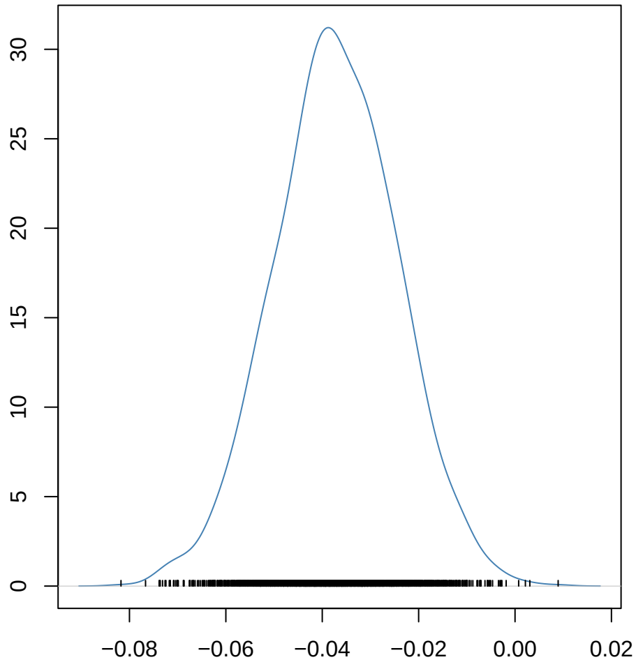
propAccelDn~masdif
