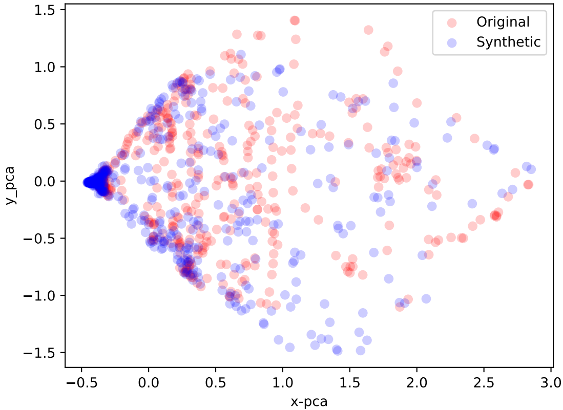
PCA plot
