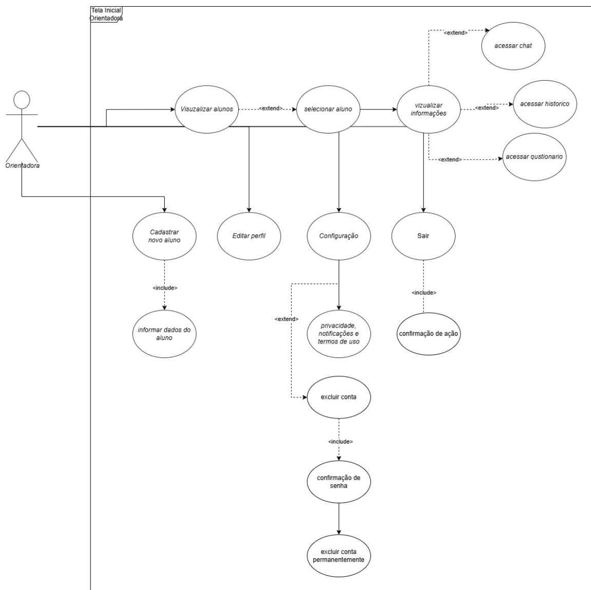
Figura 20 Diagrama de casos de uso 0.1
