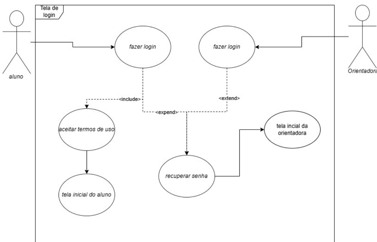
Figura 19 Diagrama de casos de uso 0.0
