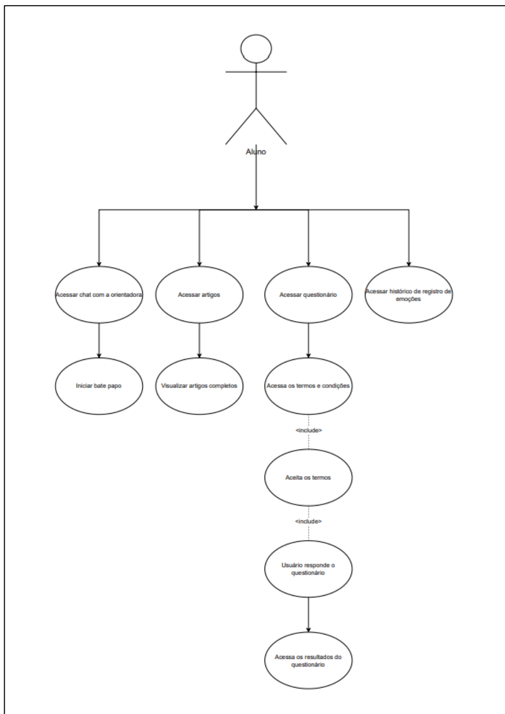
Figura 22 diagrama casos de uso 0.3
