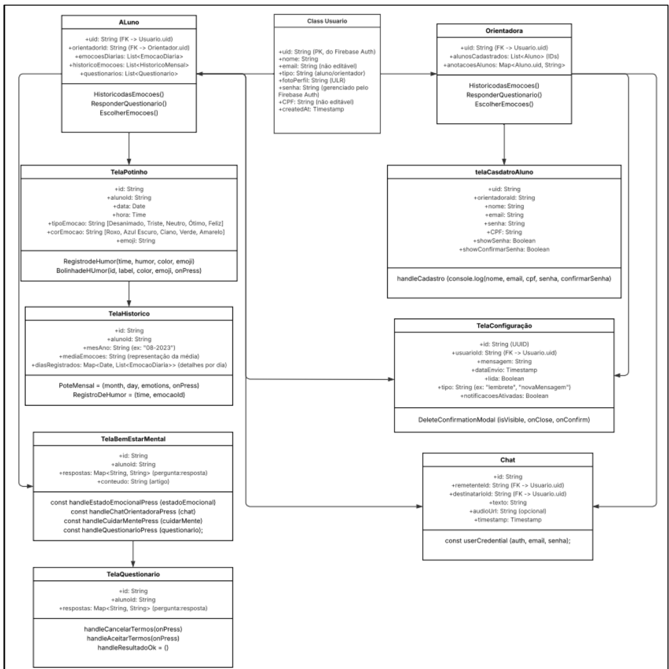
Figura 23 Diagrama de classe
