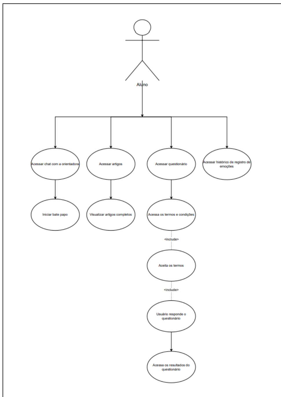
Figura 21 diagrama casos de uso 0.2
