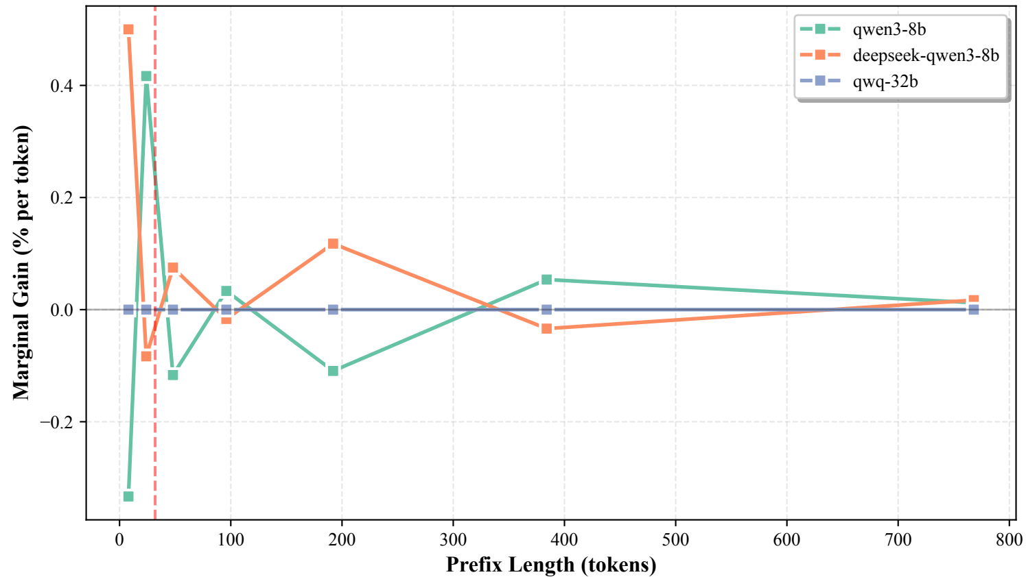
Oracle Prefix: Marginal Gain per Token
