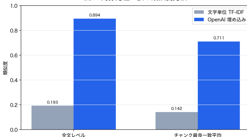
図 3: 阿弥陀経二訳の類似度比較。意味埋め込みは内容の近さを、文字単位 TF-IDF は語彙・表記差を強く反映する。
