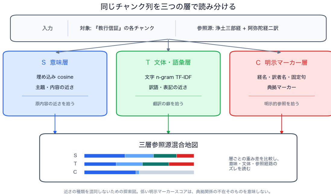
図 1: 意味・文体・典拠マーカの三層参照源混合地図の概念図。同じ対象チャンク列を、意味層、文体・語彙層、明示マーカ層の三つの指標で読み分け、層ごとの重み差から近さの種類のズレを解釈する。
