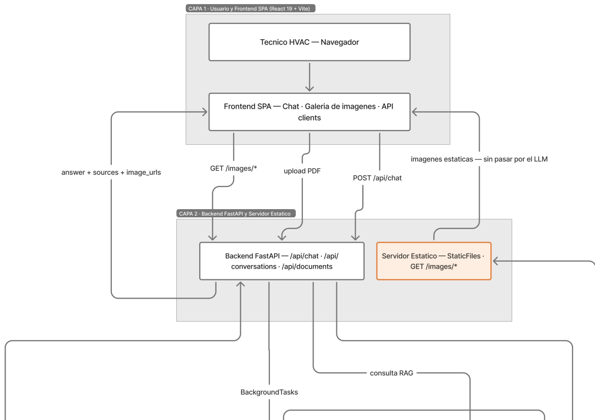
figure 4.1 Arquitectura Final del Sistema RAG para diagnóstico de HVAC. Vista 1: capas de usuario y backend. Fuente: [Elaboración propia]
