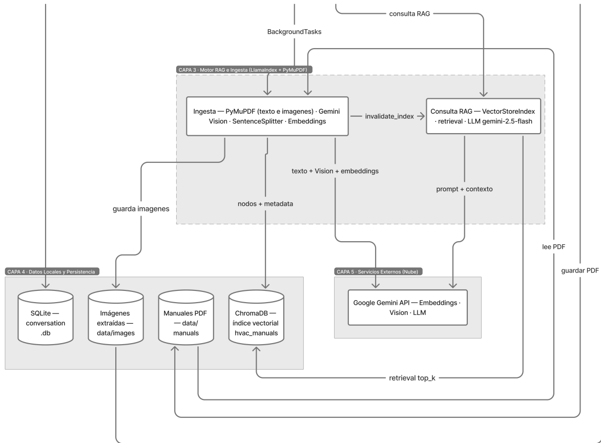
figure 4.2 Arquitectura Final del Sistema RAG para diagnóstico de HVAC. Vista 2: motor RAG, persistencia y servicios externos. Fuente: [Elaboración propia]
