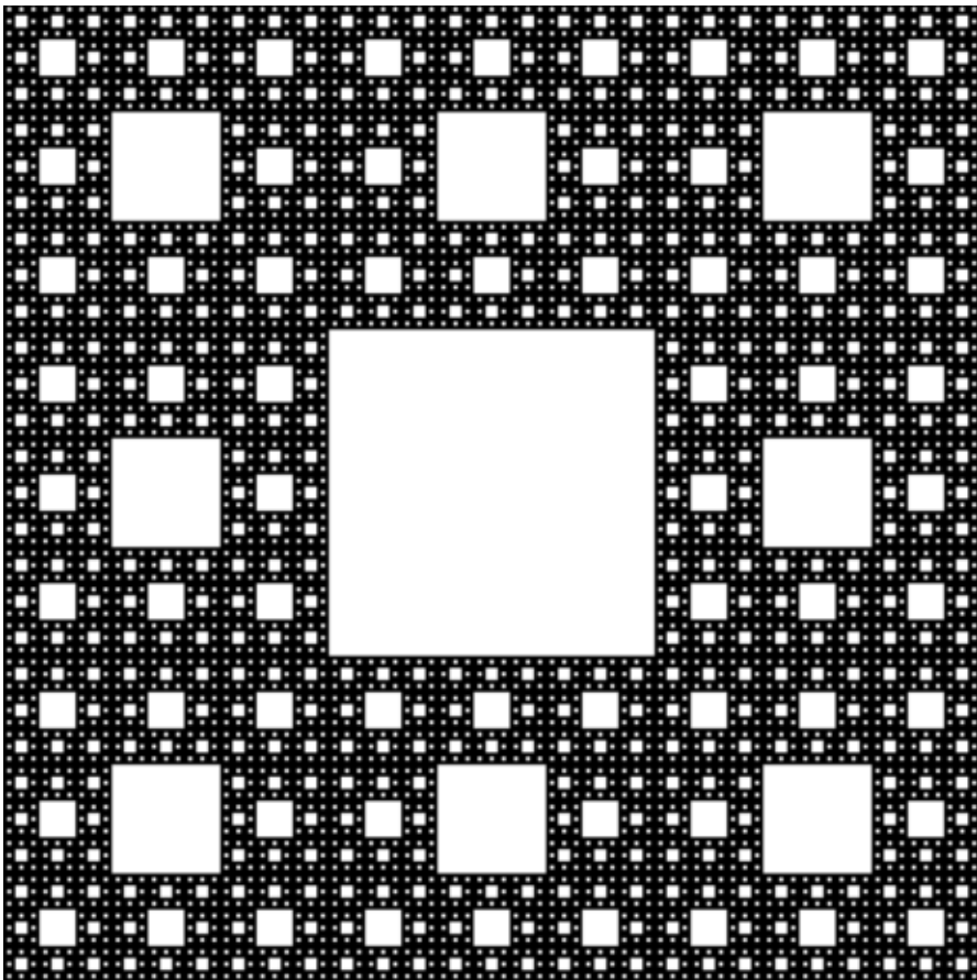
Sierpinski Carpet
