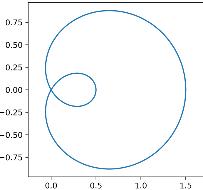
Limacon
