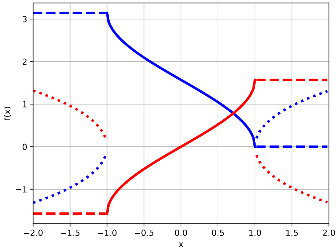
Plot2dAcosAsin, mpm
