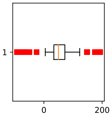
horizontal boxes
