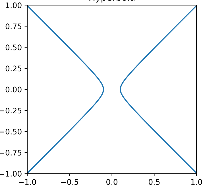
Hyperbola
