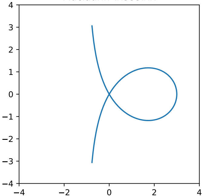
Maclaurin trisectrix
