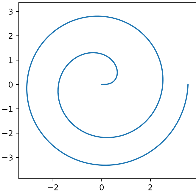
Fermat Spiral
