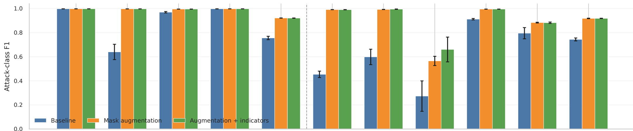
CSE-CIC-IDS2018 target test
