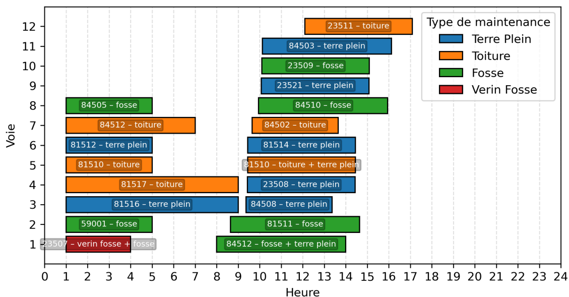
Occupation des voies journée type – site de MBC
