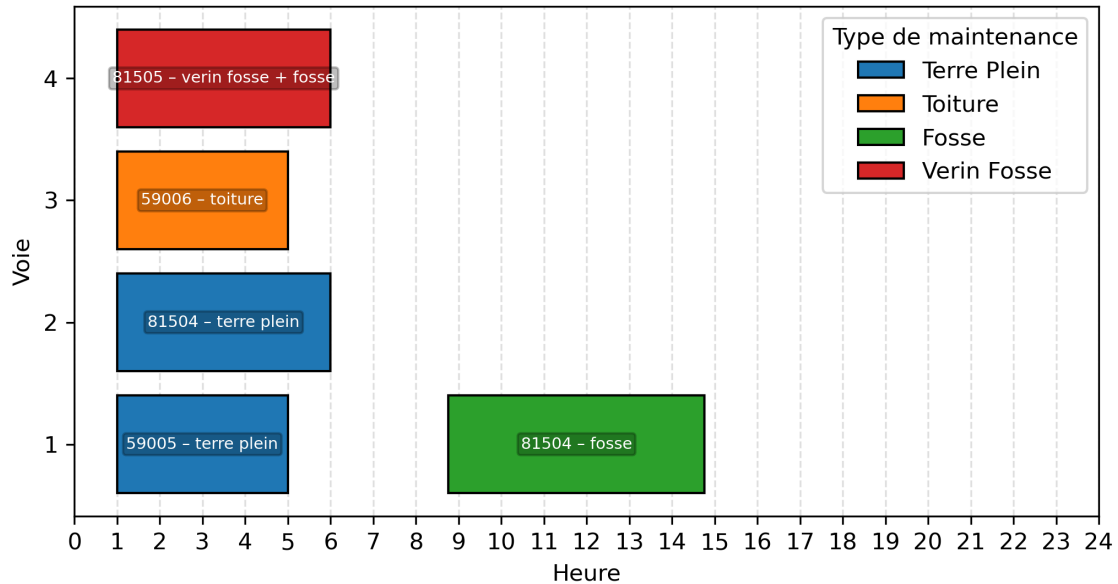
Occupation des voies journée type – site de AVG
