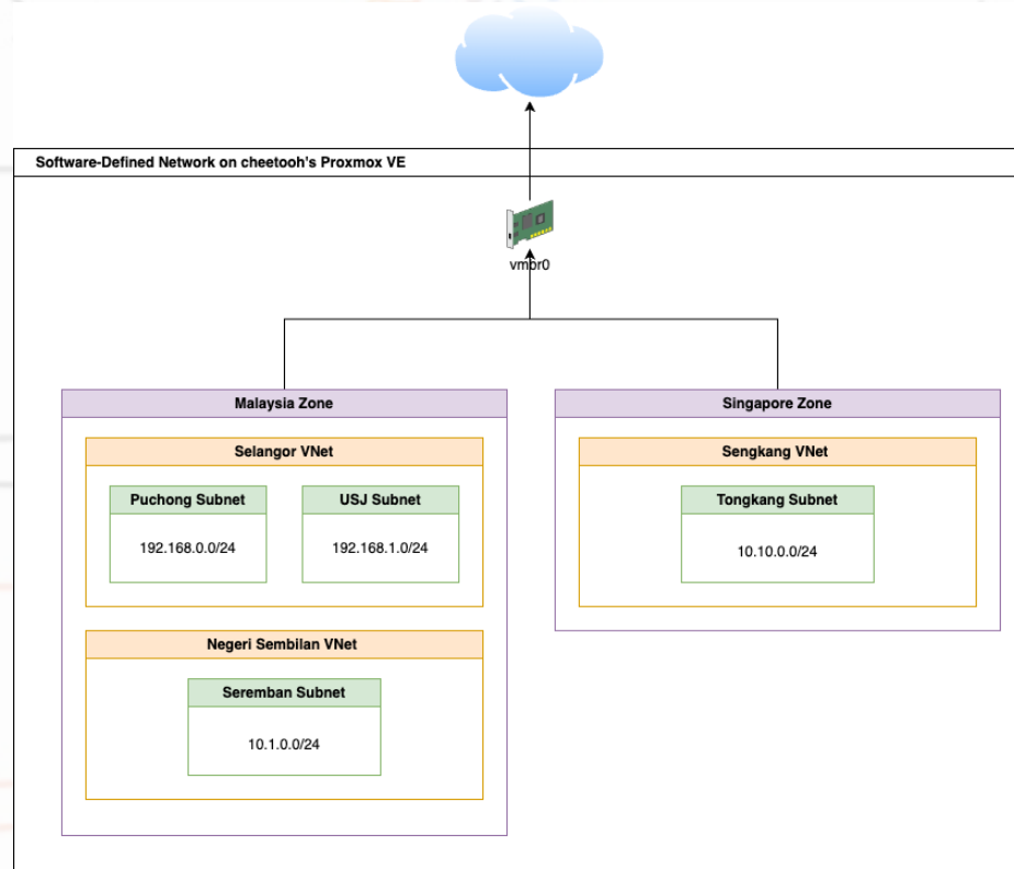
Proxmox SDN
