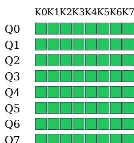
图 20 绿色 cell (i, j) = \text{block } i \text{ 的 thread } j \text{ 算 } S[i, j] = q_i \cdot k_j 。一行 8 个 thread 仍只填满 warp 的 1/4——矩阵再小也改不了 blockDim < 32 的 lane 浪费。
