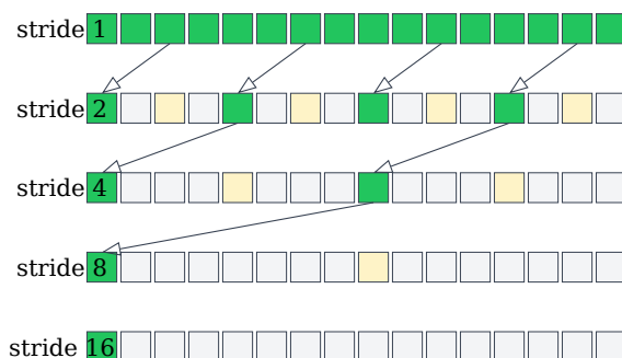
图 8 Interleaved addressing 对比 : 活跃 lane 间隔分布 , warp 内 lane 部分 active、部分 idle ——但 ncu 显示 \text{issued}/32 = 32 ( 是 predicated , 不是 divergence )。真正的差别是访问模式导致的 bank conflict pattern。
