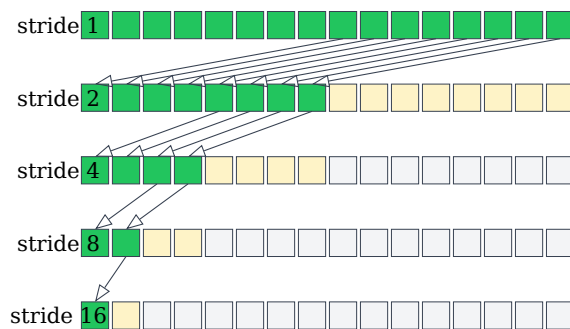
图 15 block 版 mean/var tree 同一模式：每轮活跃 lane 连续但数量减半。H = 256 时 smem conf. = 0 ——源码里第一轮 offset = 128 可能触发 32-way bank conflict，但规约步数少、block 仅 64 个，ncu 累积不到可观测 conflict；不能从代码结构 alone 断言 bench 里一定有 conflict 。
