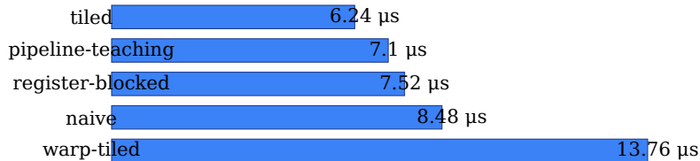
图 11 time ( \mu s) 排序: tiled smem 复用 win; warp-tilted 结构复杂度在小 N 下反噬。
