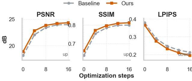
图 4. 前馈回归器消融的早期收敛对比。图中从左到右分别给出了插入后前 16 次局部优化内的 PSNR、SSIM 和 LPIPS 均值曲线，用于补充展示 Baseline 与 Ours 在早期阶段的收敛差异。
