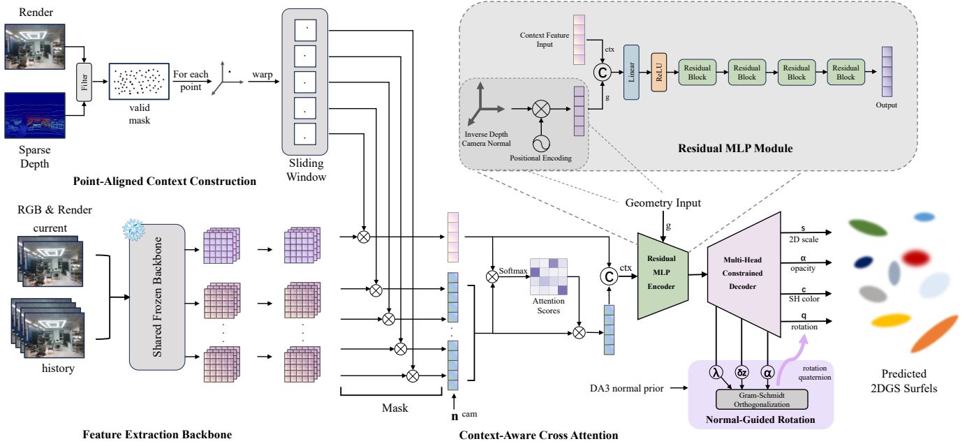
图 2. 上下文感知前馈高斯回归器结构。网络首先在滑动窗口内对有效候选种子构造逐点对齐的上下文，并通过冻结的共享主干提取当前帧与历史帧的图像-渲染特征；随后，跨注意力模块汇聚多视图外观信息，并与逆深度、DA3 法线和位置编码等几何先验一起输入残差 MLP 编码器；最后，多头约束解码器预测完整的 2DGS surfel 属性 (\mu, s, \alpha, c, q) ，其中法线引导的旋转分支通过 Gram-Schmidt 正交化构造几何一致的朝向。
