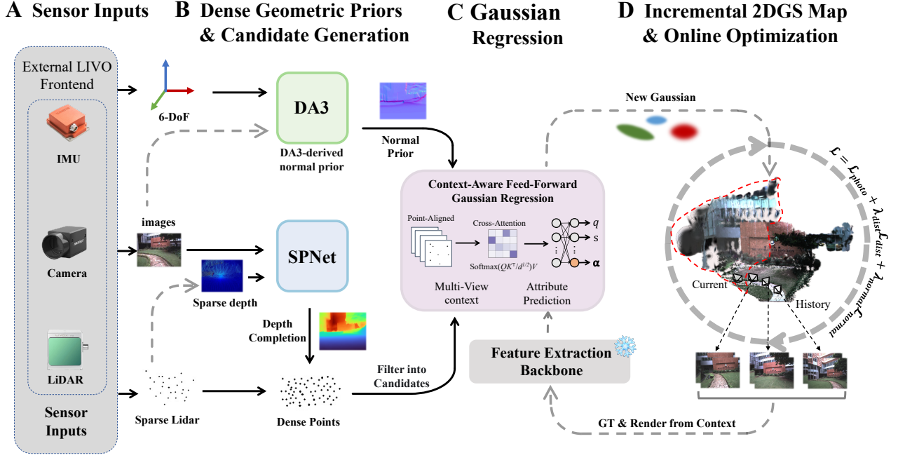
图 1. 系统整体流程。(A) 外部 LiDAR-惯导-视觉前端提供同步的 RGB 图像、LiDAR 观测、IMU 信息和相机位姿。(B) 系统利用 SPNet 深度补全和 DA3 法线估计生成稠密几何先验，并与 LiDAR 点共同形成欠重建区域的初始点。(C) 对于每个候选点，前馈高斯回归器聚合逐点对齐的多视图上下文，直接预测 2DGS surfel 属性。(D) 预测得到的新 surfel 被插入增量地图后，再结合在线优化进一步更新；同时，当前地图的渲染结果继续作为后续插点的上下文输入。
