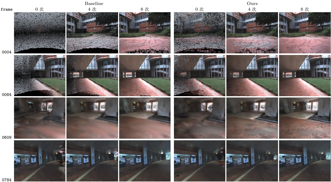
图 4. 前馈回归器消融的可视化结果。展示代表帧 train_0004、train_0084、train_0609 与 train_0784 在 0、4、8 次对当前帧的优化后的结果；每行左三列为 Baseline，右三列为 Ours。
