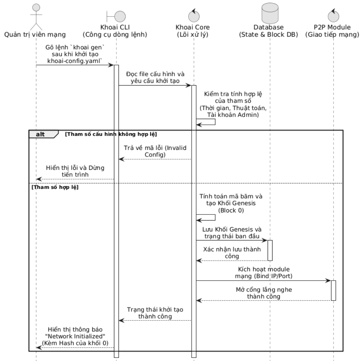
Hình 4: Sơ đồ Sequence khởi tạo mạng lưới Khoai Chain
