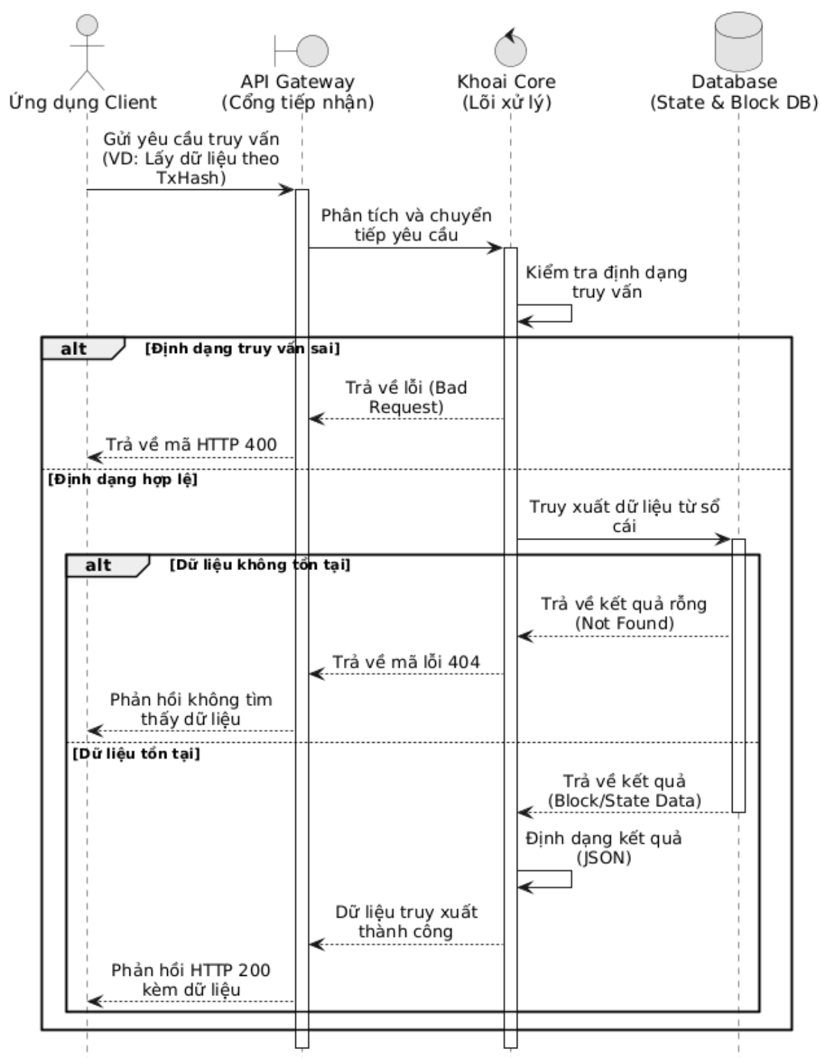
Hình 8: Sơ đồ Sequence truy vấn sổ cái Khoai Chain
