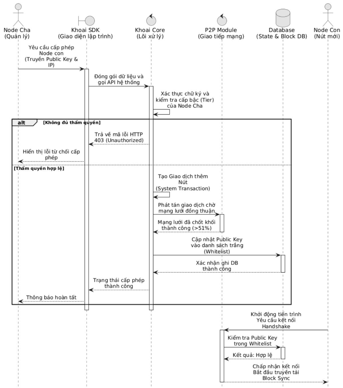
Hình 5: Sơ đồ Sequence tạo Node mới Khoai Chain
