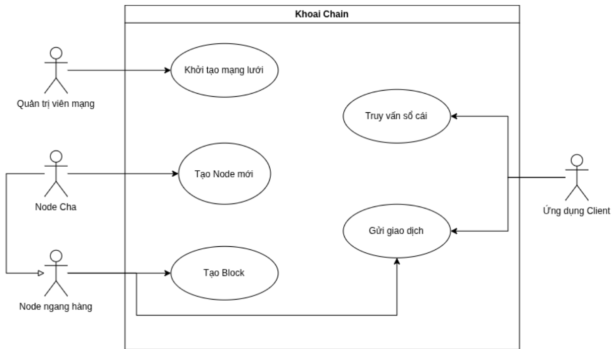
Hình 3: Sơ đồ Use Case mạng lưới Khoai Chain
