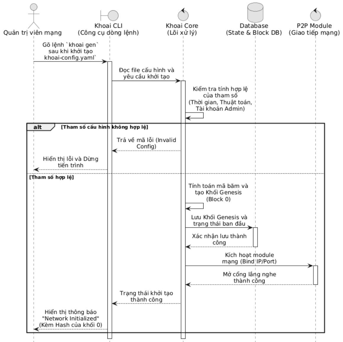
Hình 3.2: Sơ đồ trình tự khởi tạo mạng lưới Khoai Chain
