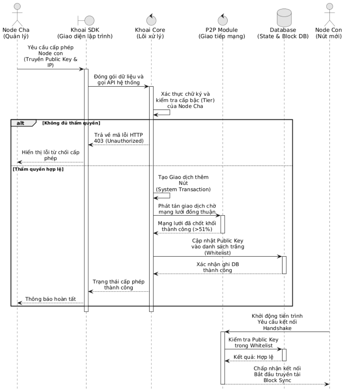
Hình 3.3: Sơ đồ trình tự tạo nút mới Khoai Chain
