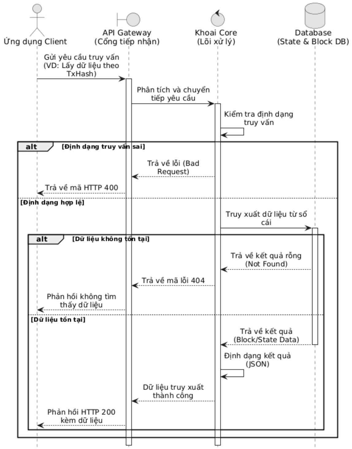
Hình 3.6: Sơ đồ trình tự truy vấn sổ cái Khoai Chain
