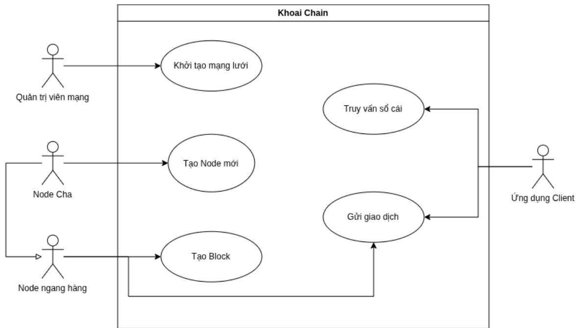
Hình 3.1: Sơ đồ trường hợp sử dụng mạng lưới Khoai Chain
