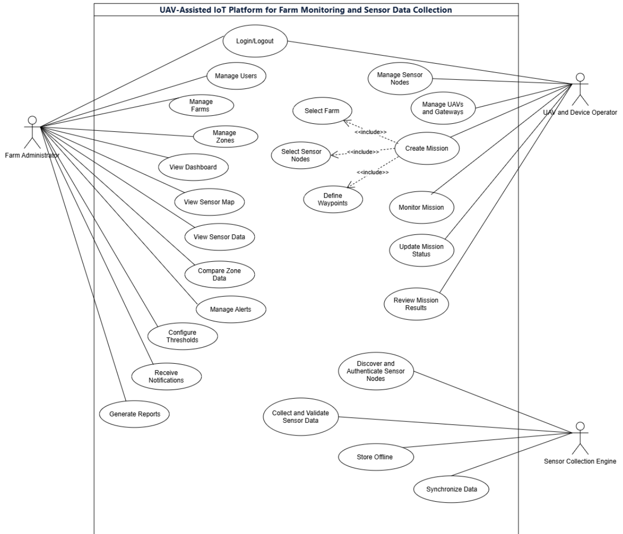
Hình 1: Use Case Diagram
