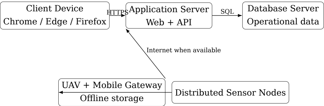
Hình 4.6: Deployment Diagram
