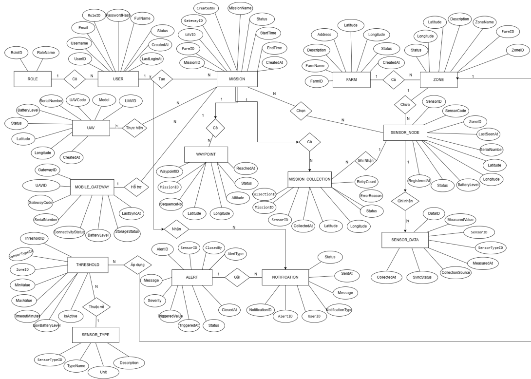
Hình 1: ERD
