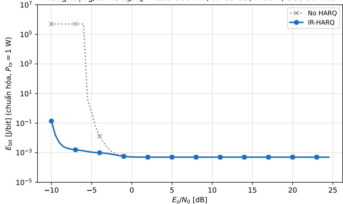
Năng lượng/bit vs E_s/N_0 -- LEO 600 km, K=15 dB, MCS A, SCS 30 kHz
