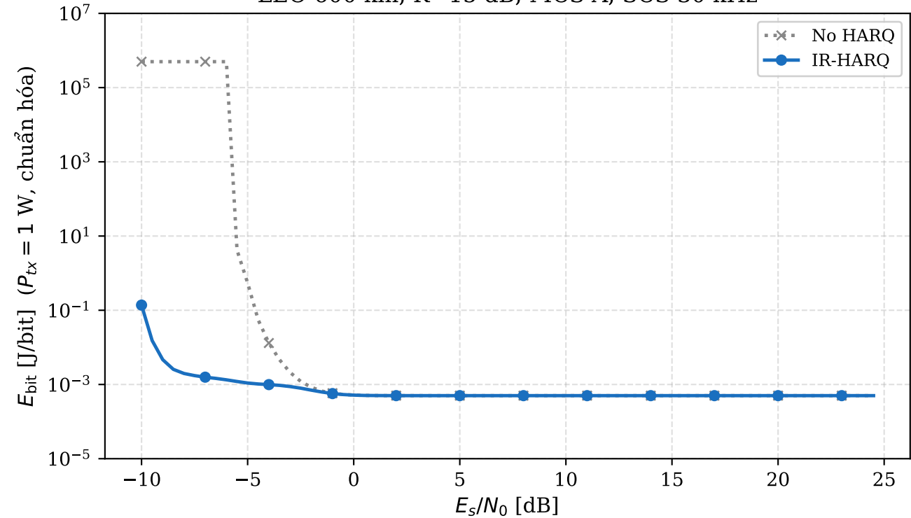
Năng lượng/bit vs E_s/N_0 LEO 600 km, K=15 dB, MCS A, SCS 30 kHz
