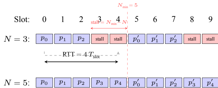
Hình 2.1 Sơ đồ thời gian pipeline HARQ (ví dụ minh họa: \text{RTT} = 4 T_{\text{slot}} , N_{\min} = 5 ). Hàng N = 3 < N_{\min} : 2 slot stall sau mỗi 3 slot hữu ích – util = 3/5 = 60\% . Hàng N = 5 = N_{\min} : pipeline đầy liên tục – util = 100%. Trong NTN thực (LEO 600 km, SCS 30 kHz): \text{RTT} \approx 12,88 ms \approx 26 T_{\text{slot}} , N_{\min} = 27 .
