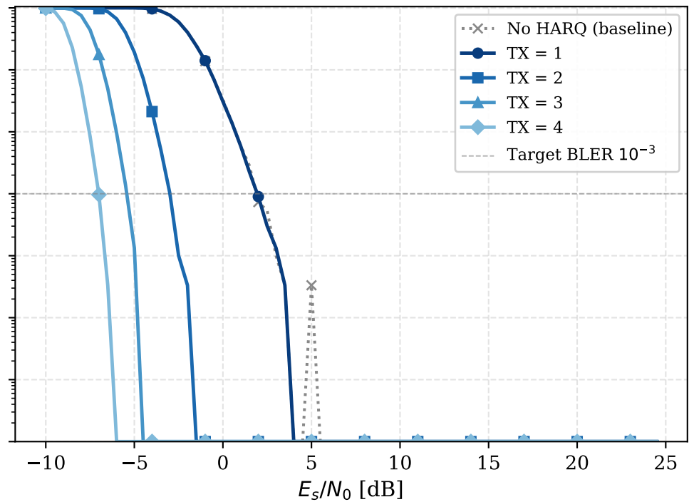
(b) IR-HARQ
