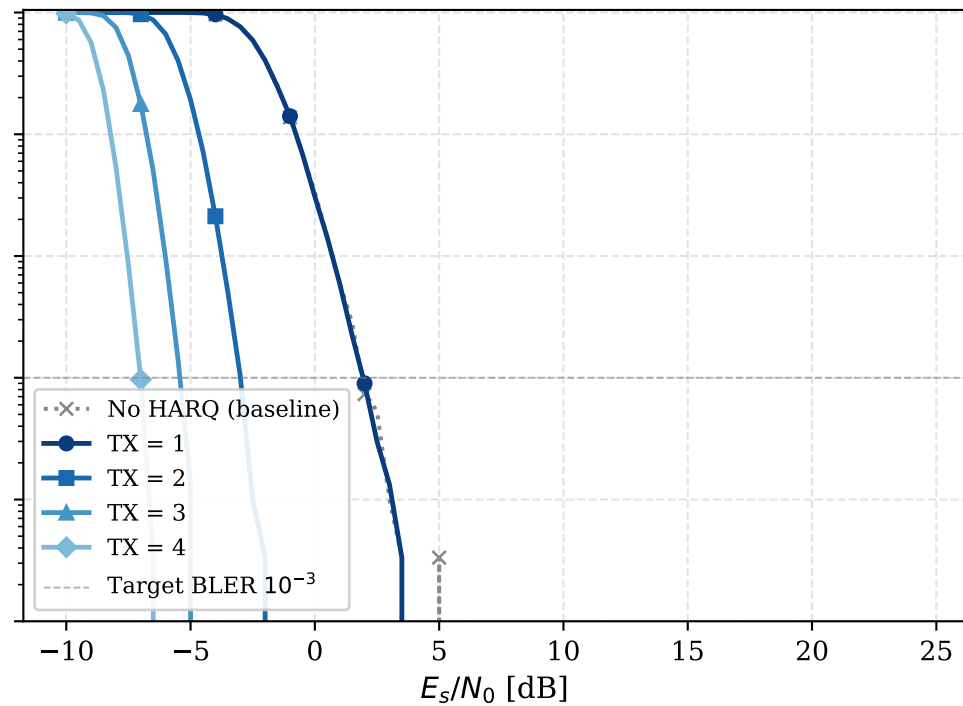
(b) IR-HARQ
