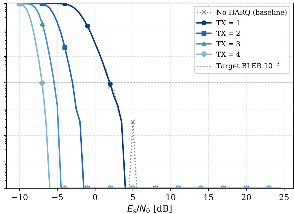
(b) IR-HARQ
