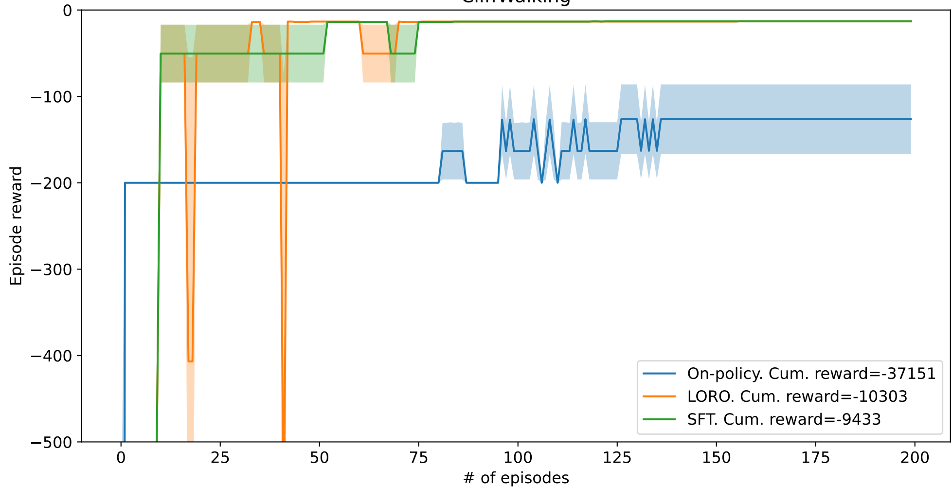
CliffWalking
