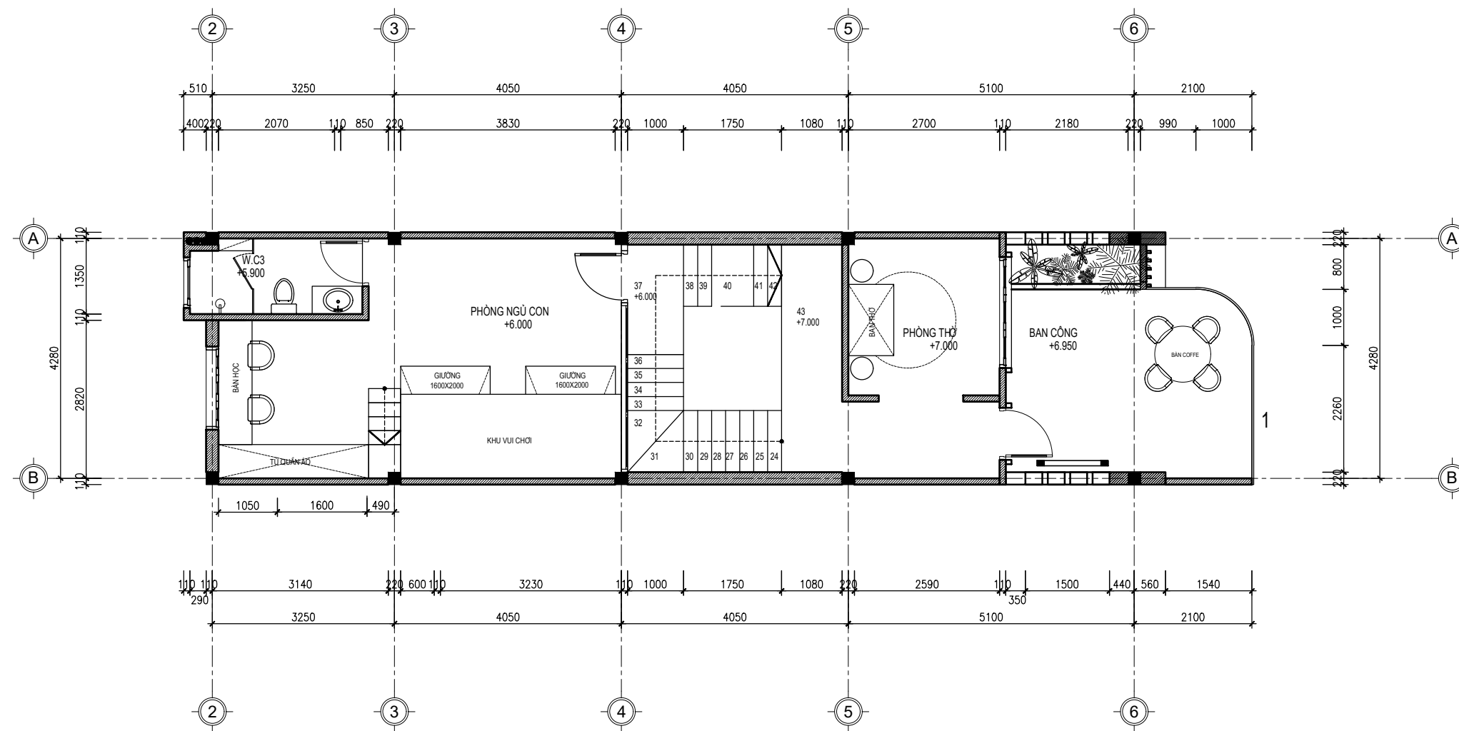
MẶT BẰNG TẦNG 3
