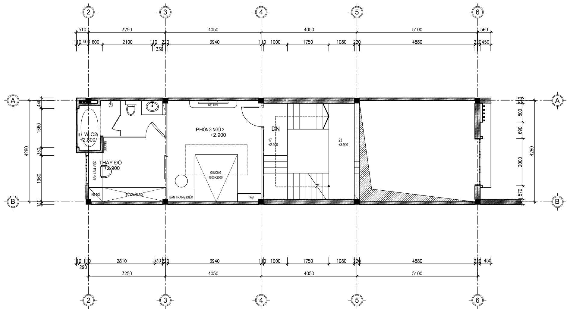
MẶT BẰNG TẦNG 2
