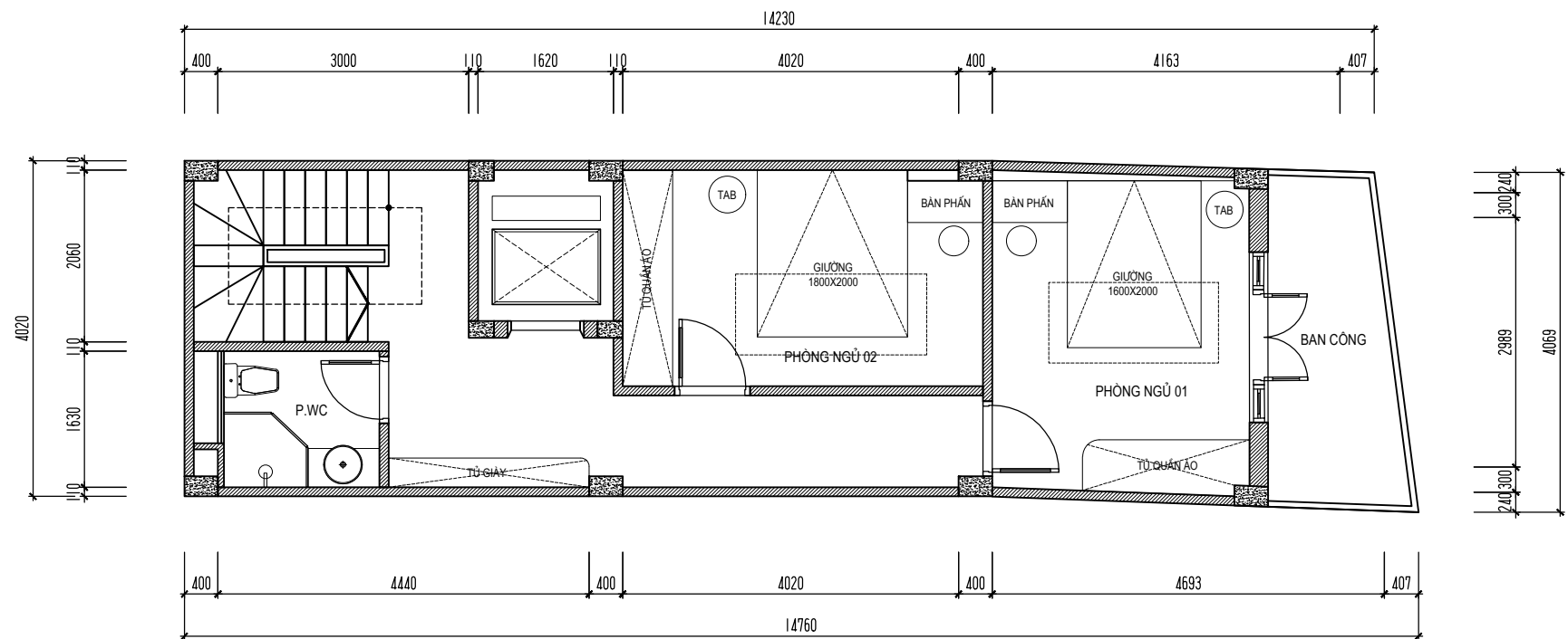
PHƯƠNG ÁN BỐ TRÍ MẶT BẰNG TẦNG 6
