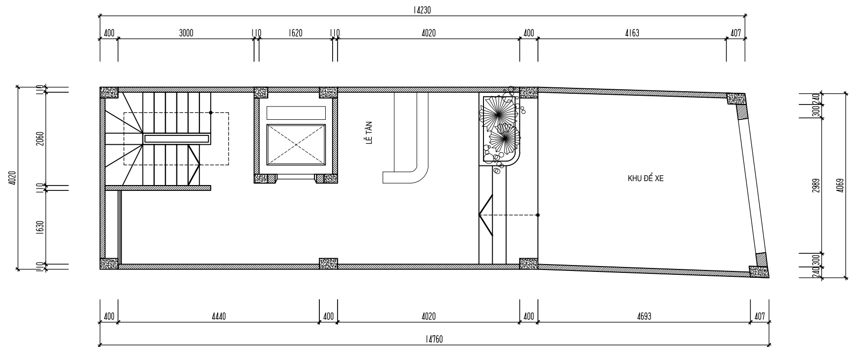
PHƯƠNG ÁN BỐ TRÍ MẶT BẰNG TẦNG 1
